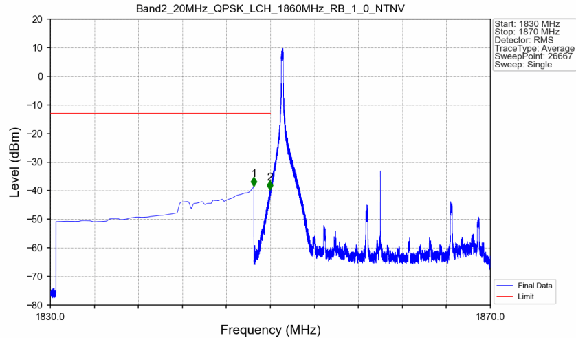
Band2_20MHz_QPSK_LCH_1860MHz_RB_1_0_NTNV
