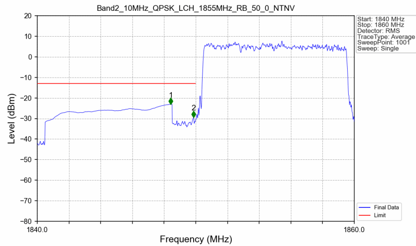
Band2 10MHz QPSK LCH 1855MHz RB 50 0 NTNv
