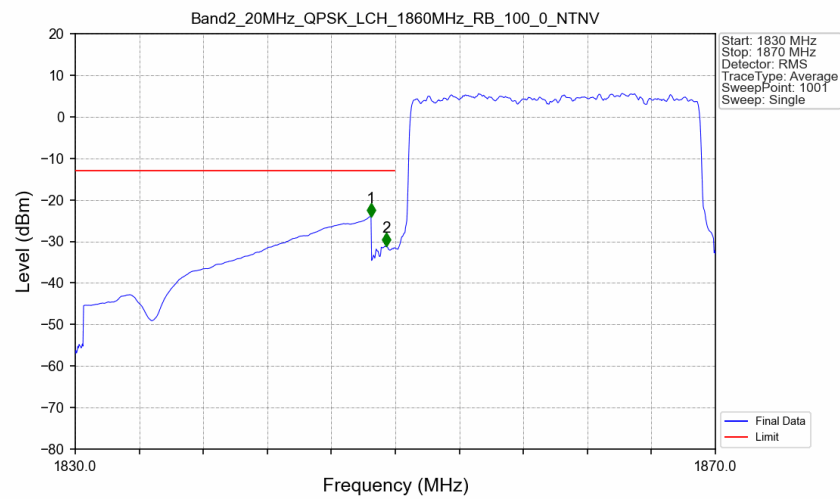
Band2 20MHz QPSK LCH 1860MHz RB 100 0 NTN
