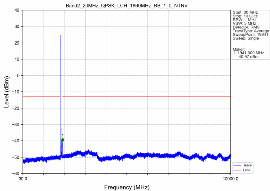
Band2_20MHz_QPSK_LCH_1860MHz_RB_1_0_NTNV
