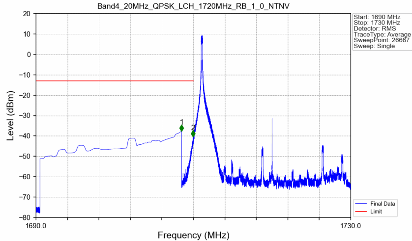
Band4_20MHz_QPSK_LCH_1720MHz_RB_1_0_NTNV
