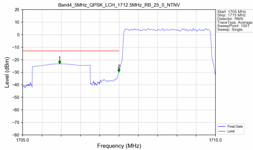
Band4 5MHz QPSK LCH 1712.5MHz RB 25 0 NTNV
