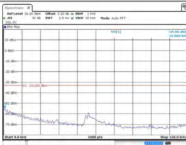
GSM850_128
