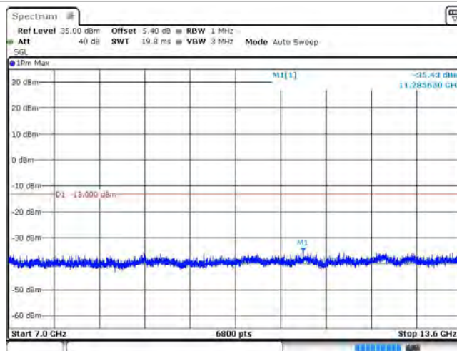
GSM1900_810
