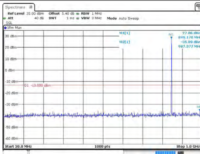
EGPRS850_251
