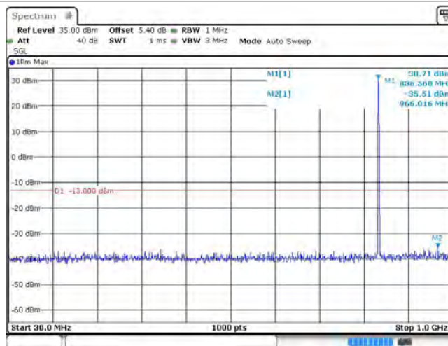
GSM850_190
