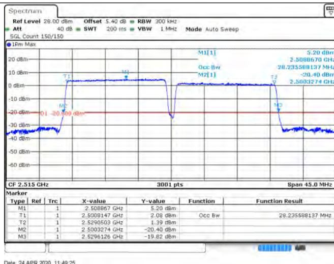
CA 7C 15+15 QPSK 21025+21175 75RB#0+75RB#0
