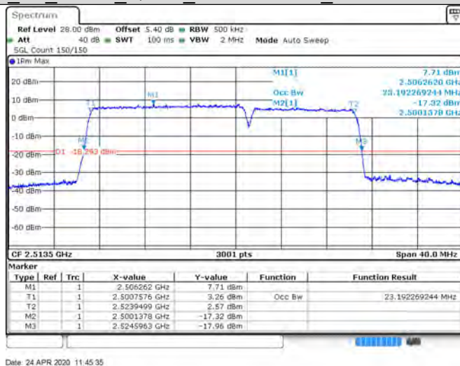
CA 7C 15+10 QPSK 21051+21171 75RB#0+50RB#0
