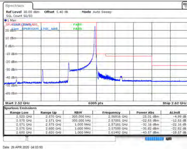
CA 7C 75RB+75RB 64QAM 21225+21375 75RB#0+75RB#0
