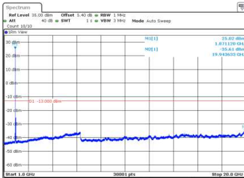
Band2-20MHz-16QAM-18900-1RB#0-Range2:1000~20000MHz
