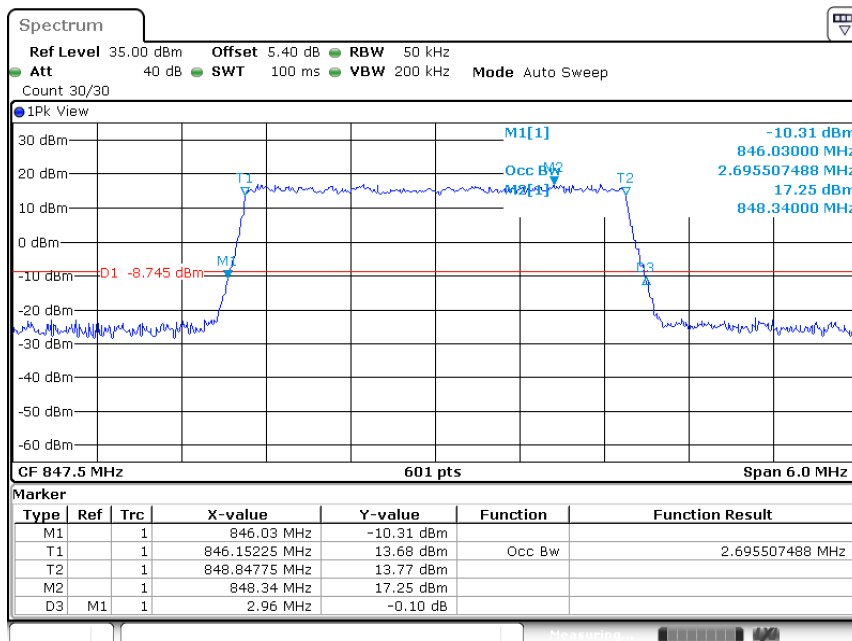
Band5-3MHz-QPSK-20635-15RB#0-2.696
