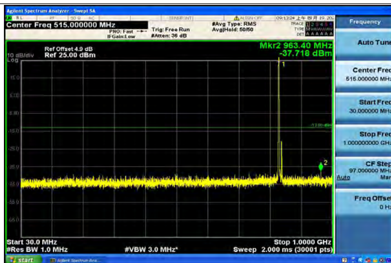
Band5-10MHz-16QAM-20525-1RB#0-Range2:1000~5000MHz
