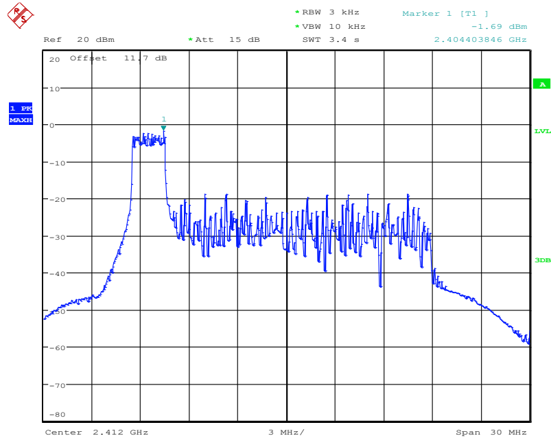
Fig.A.3.1 ANT3 802.11ax-HE20 RU26-left ch1
