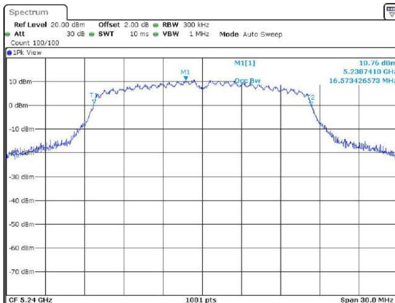
11A-CDD_Ant2_5240
