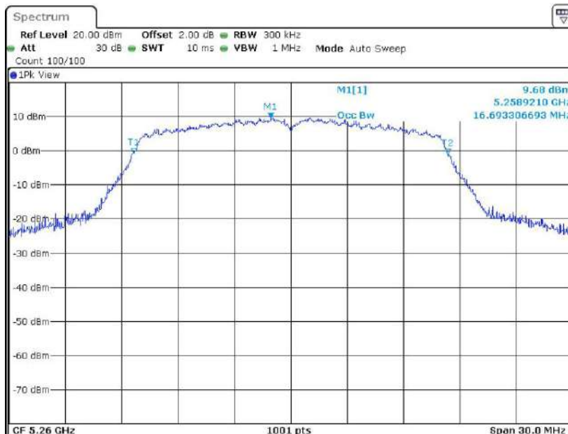
11A-CDD_Ant1_5260
