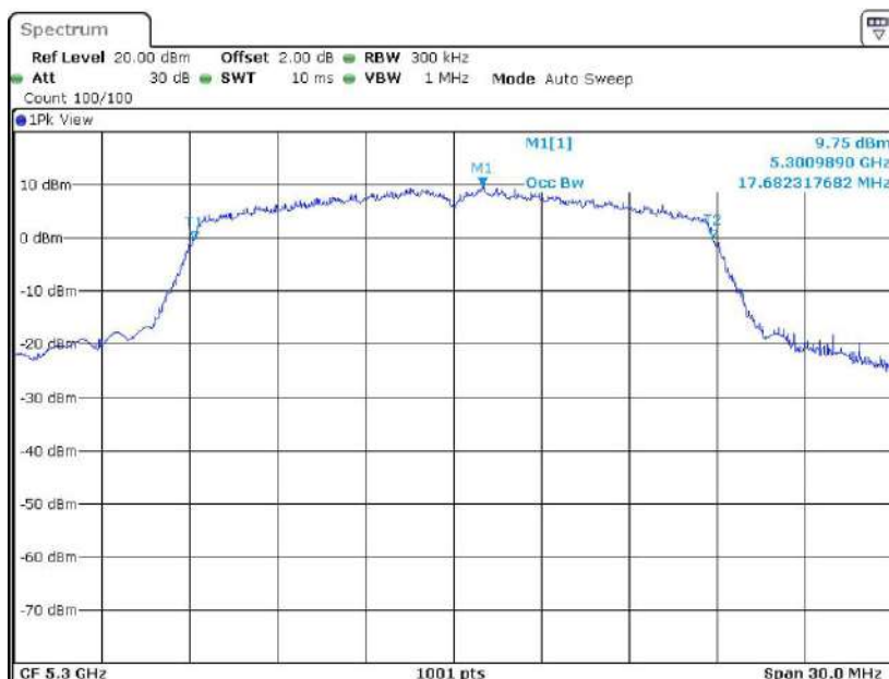
11N20MIMO Ant1 5300
