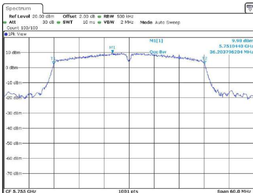
11N40MIMO Ant1 5755
