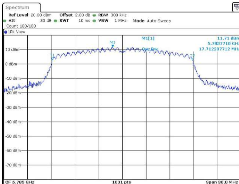
11AC20MIMO_Ant2_5785
