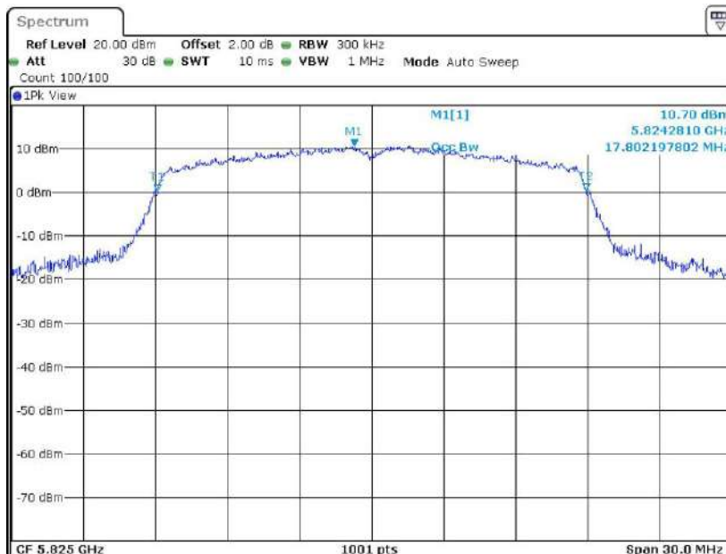
11AC20MIMO_Ant1_5825
