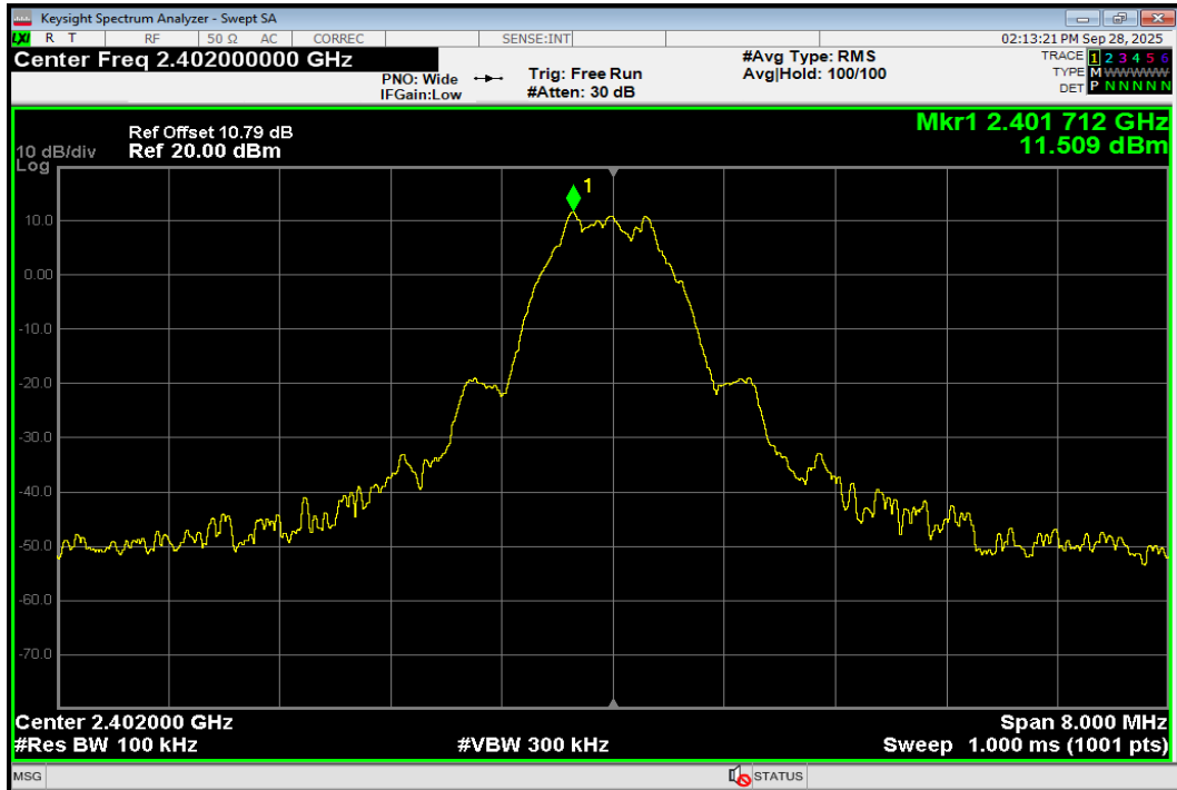
Band Edge BLE (1M) 2402MHz Emission
