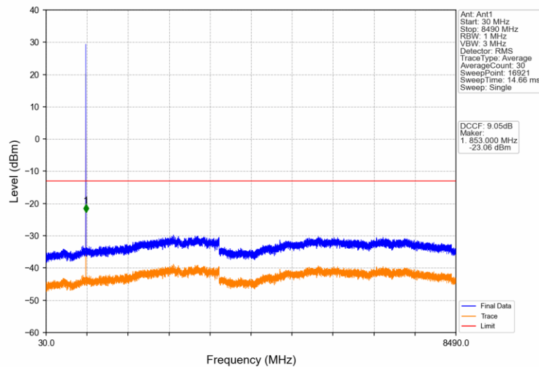
GSM850_GPRS_HCH_848.8MHz_1 TX Slot_NTNV
