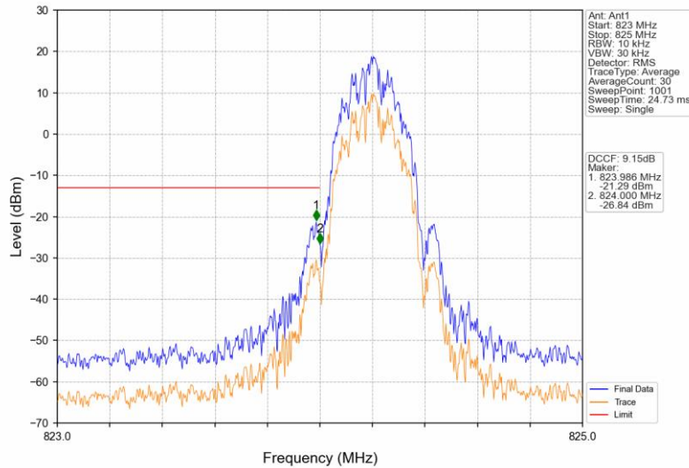
GSM850_EGPRS_LCH_824.2MHz_1 TX Slot_NTNV
