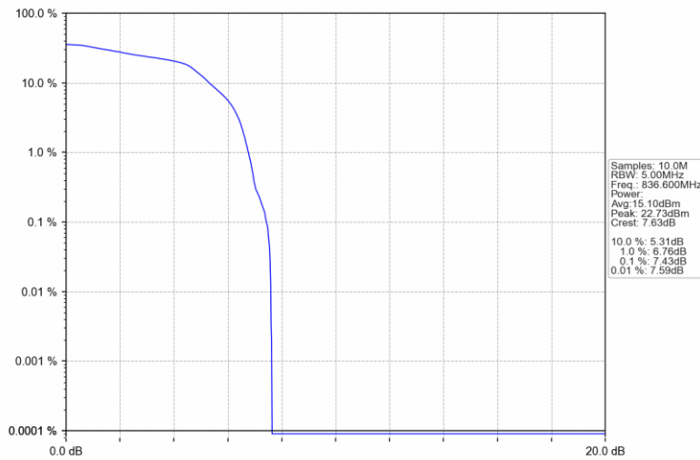
GSM850_EGPRS_MCH_836.6MHz_4 TX Slots_NTNV
