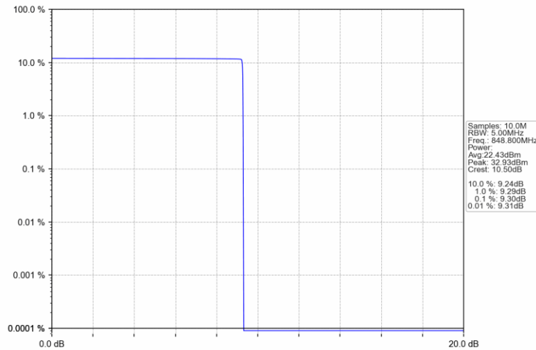
GSM850_GSM_HCH_848.8MHz_GSM_NTNV
