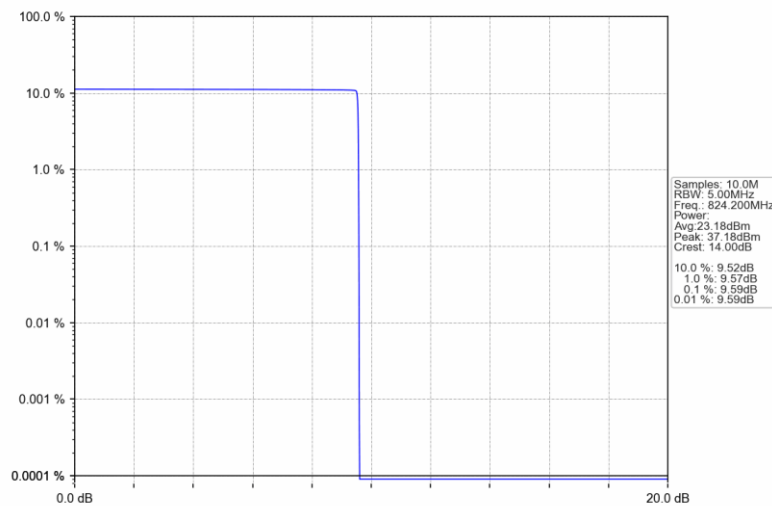
GSM850_GPRS_LCH_824.2MHz_4 TX Slots_NTNV
