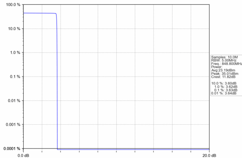
GSM850_GPRS_HCH_848.8MHz_4 TX Slots_NTNV
