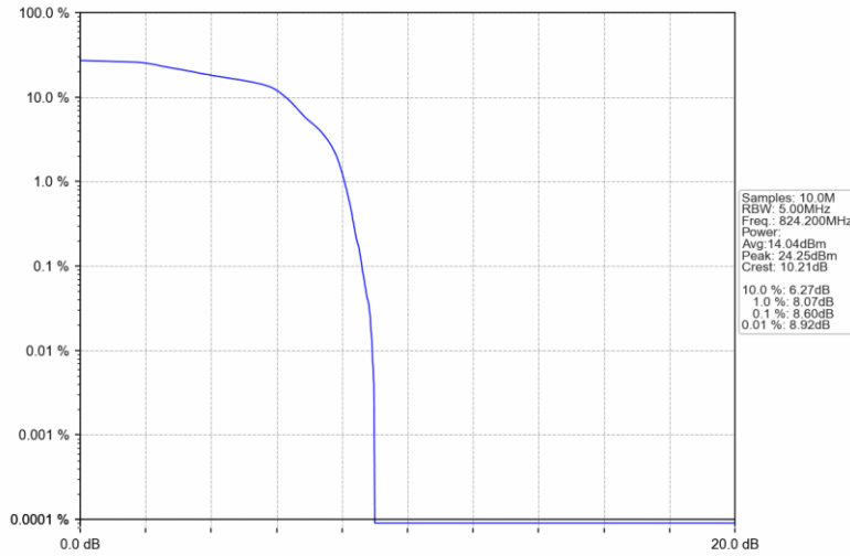
GSM850_EGPRS_LCH_824.2MHz_4 TX Slots_NTNV
