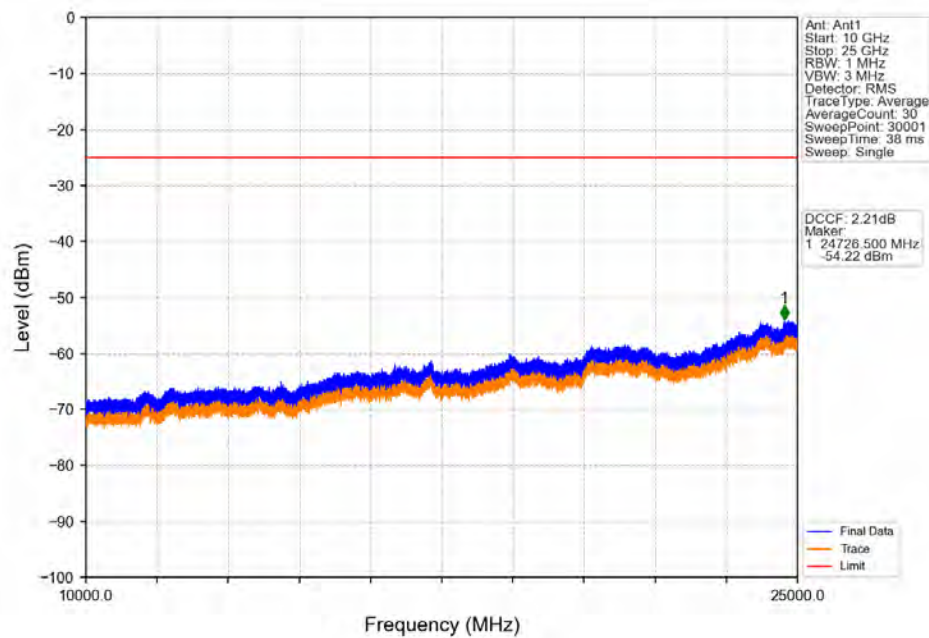
Band38_10MHz_QPSK_MCH_2595MHz_RB_1_0_NTNV
