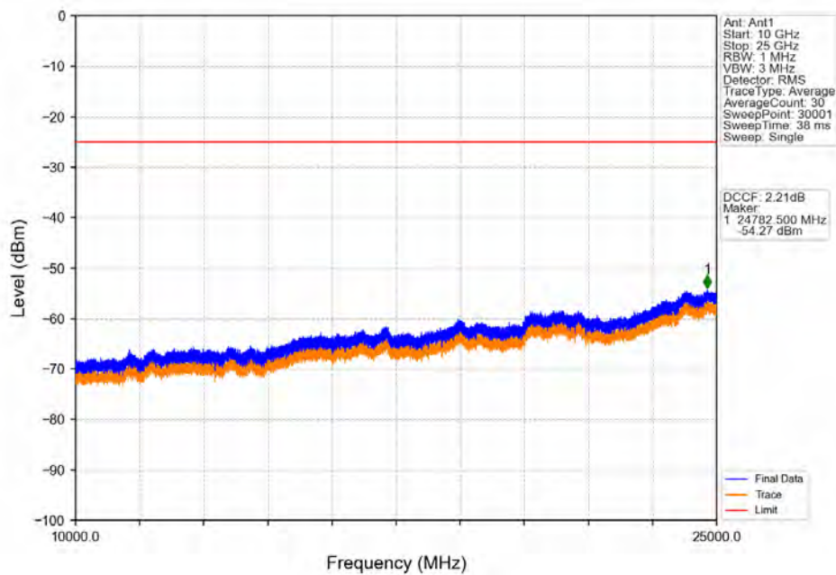
Band41_5MHz_QPSK_MCH_2593MHz_RB_1_0_NTNV
