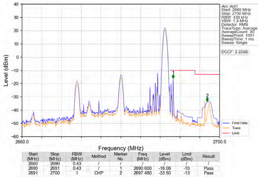
Band41_20MHz_QPSK_HCH_2680MHz_RB_1_99_NTNV
