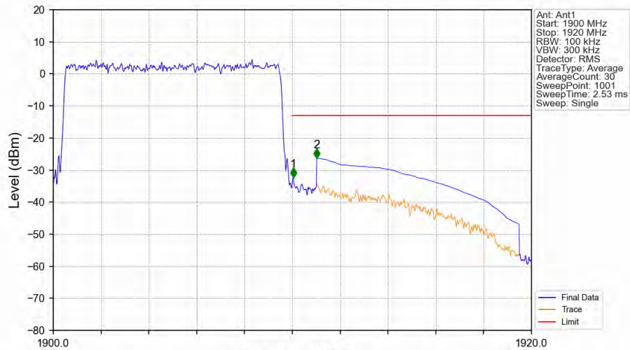
Band2_10MHz_16QAM_HCH_1905MHz_RB_50_0_NTNV
