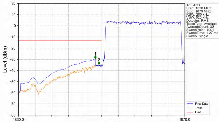
Band2_20MHz_QPSK_LCH_1860MHz_RB_100_0_NTNV
