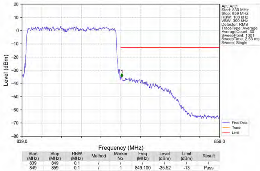
Band5_10MHz_QPSK_HCH_844MHz_RB_50_0_NTNV
