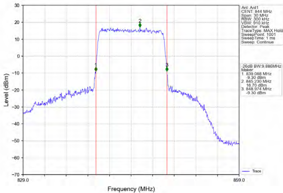
Band5_10MHz_QPSK_HCH_844MHz_RB_50_0_NTNV
