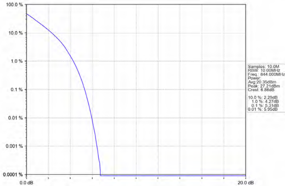
Band5_10MHz_QPSK_HCH_844MHz_RB_50_0_NTNV
