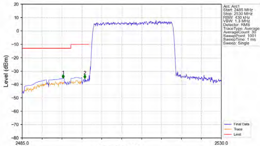
Band7_20MHz_QPSK_LCH_2510MHz_RB_100_0_NTNV
