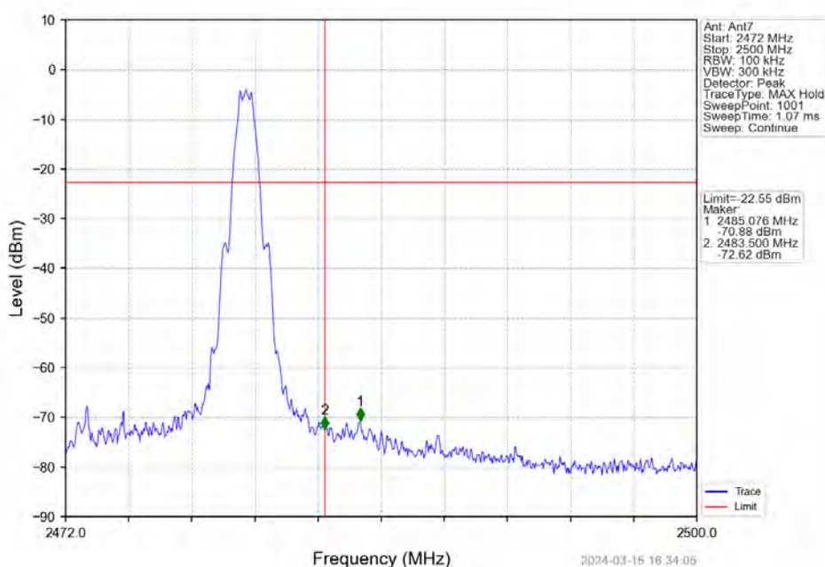
1M_HCH_2480MHz_Ant7_NTNV
