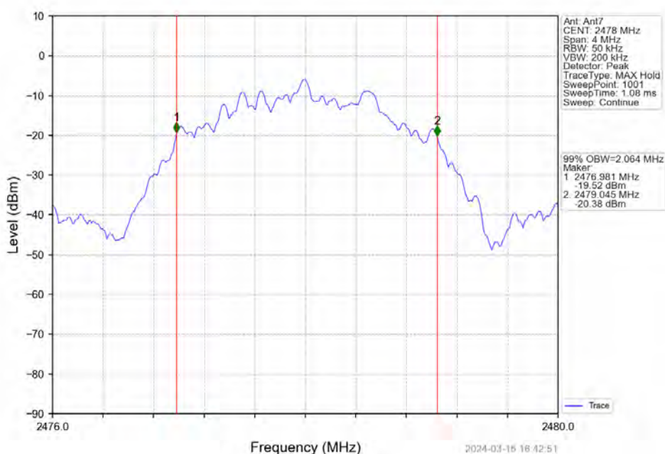
2M_HCH_2478MHz_Ant7_NTNV
