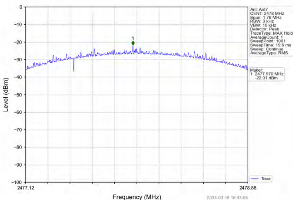
2M_HCH_2478MHz_Ant7_NTNV
