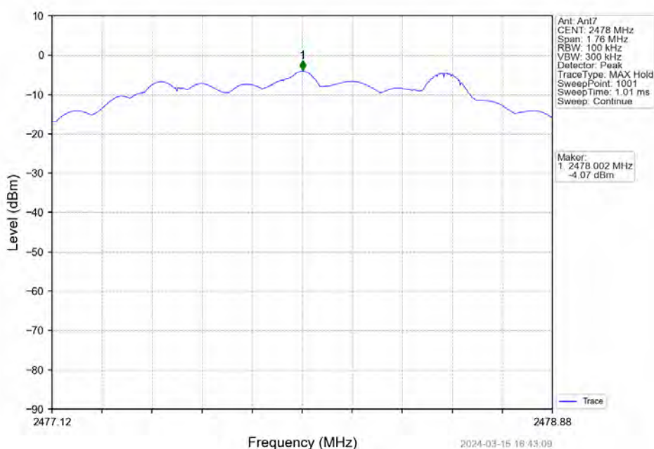
2M_HCH_2478MHz_Ant7_NTNV
