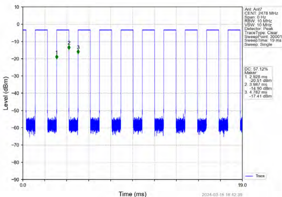
2M_HCH_2478MHz_Ant7_NTNV
