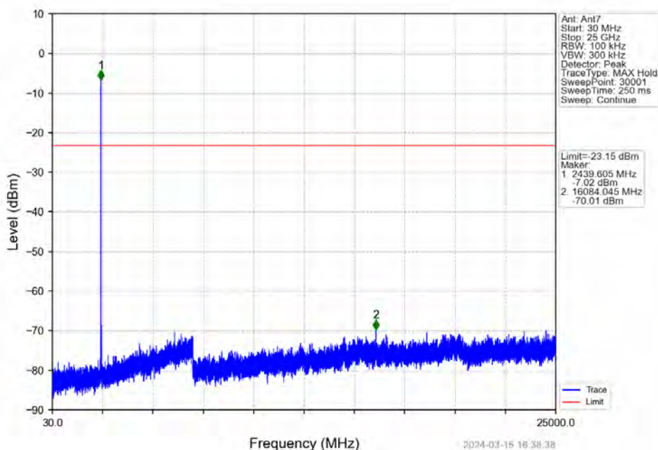
2M_MCH_2440MHz_Ant7_NTNV
