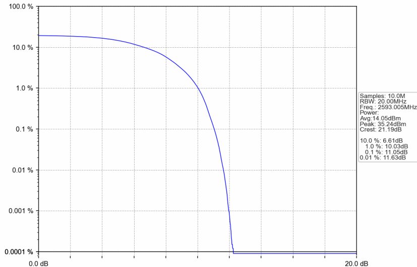
n41_15kHz_SISO_NTNV_40MHz_DFT-s-OFDM_PI/2_BPSK_2593.005MHz_Outer_Full
