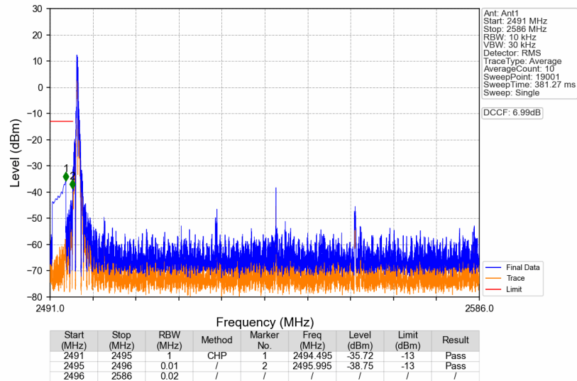
n41_30kHz_SISO_NTNV_90MHz_DFT-s-OFDM PI/2 BPSK_2541MHz_Edge_1RB_Left
