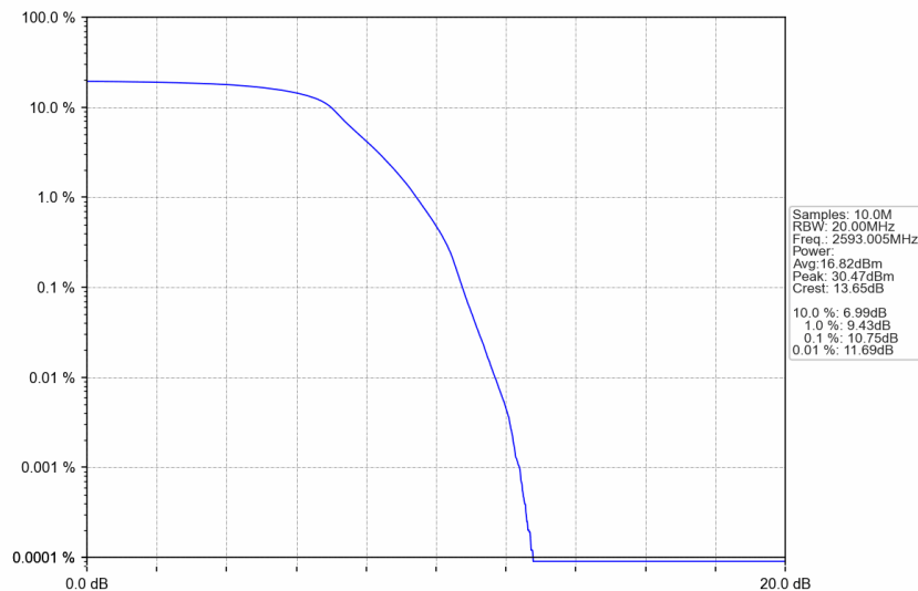
n41_15kHz_SISO_NTNV_20MHz_DFT-s-OFDM_PI/2_BPSK_2593.005MHz_Outer_Full
