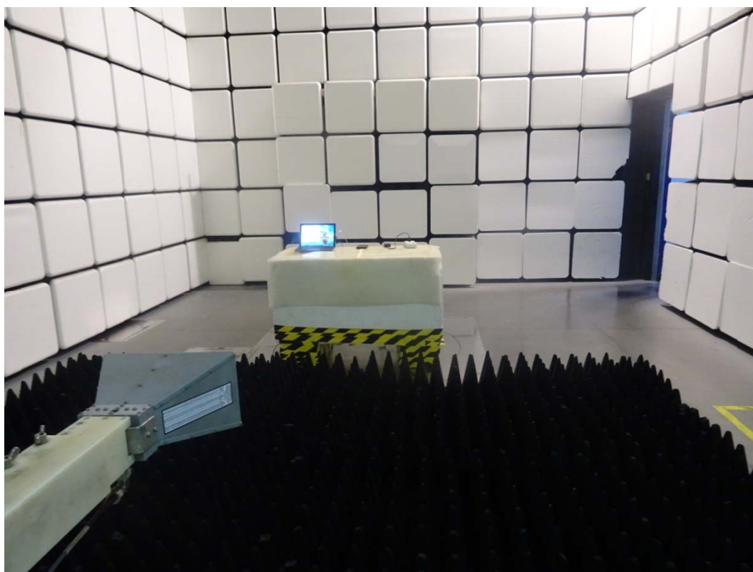
1GHz-18GHz
