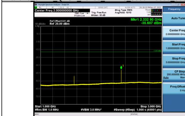
Band13 10MHz QPSK 23230 1RB#0 1000~3000 1000~3000
