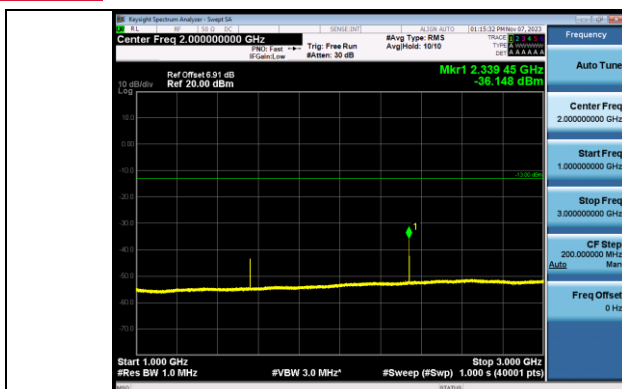
Band13 5MHz QPSK 23230 1RB#0 1000~3000 1000~3000
