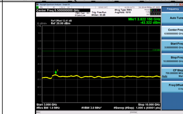
Band13 10MHz QPSK 23230 1RB#0 3000~10000 3000~10000
