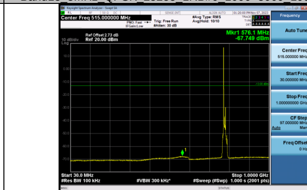
Band13 10MHz QPSK 23230 1RB#0 30~1000 30~1000
