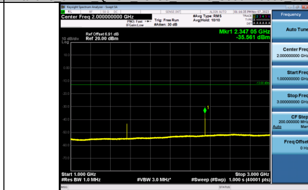
Band13 5MHz QPSK 23255 1RB#0 1000~3000 1000~3000
