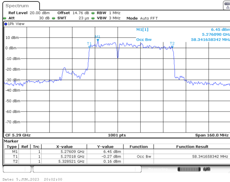
11BE80MIMO_Ant18_5290_Puncturing 20M_1
