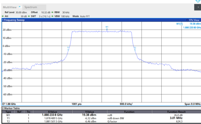
Band2-5MHz-QPSK-18900-25RB#0
