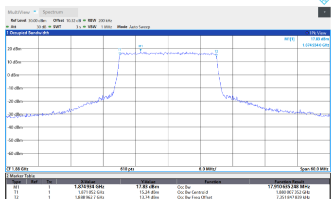
Band2-20MHz-16QAM-18900-100RB#0
