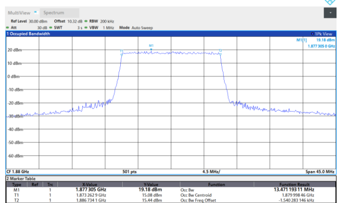
Band2-20MHz-16QAM-18900-100RB#0
