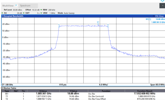
Band2-20MHz-QPSK-18900-100RB#0
