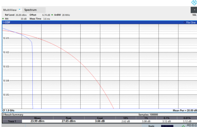
Band2-20MHz-QPSK-19100-1RB#0
