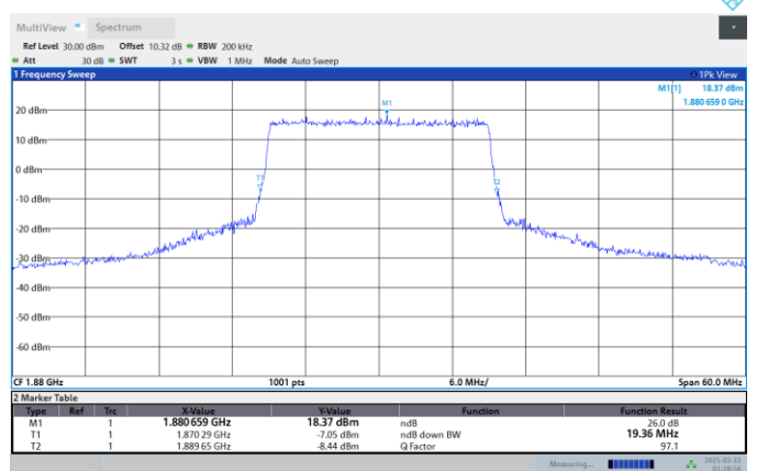
Band2-20MHz-16QAM-18900-100RB#0
