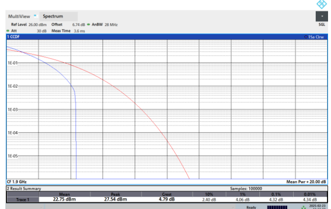
Band2-20MHz-QPSK-19100-100RB#0
