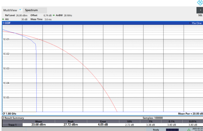
Band2-20MHz-QPSK-19100-1RB#0
