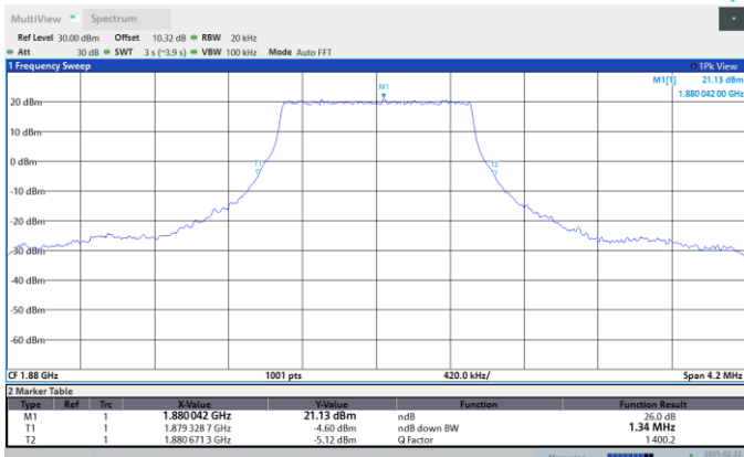
Band2-3MHz-QPSK-18900-15RB#
