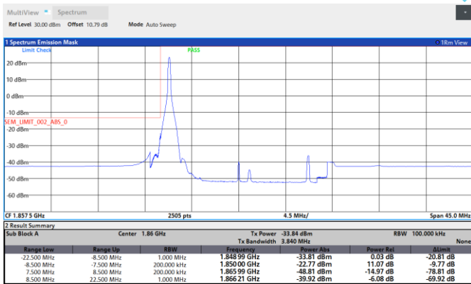
Band2-15MHz-64QAM-19125-1RB#74
