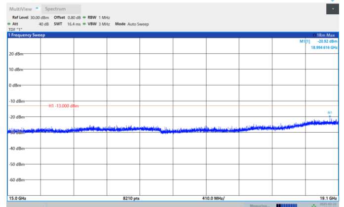
Band2-3MHz-QPSK-19185-1RB#0- Range:15000MHz~19100MHz
