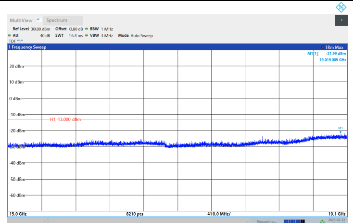
Band2-5MHz-QPSK-18625-1RB#0- Range:15000MHz~19100MHz
