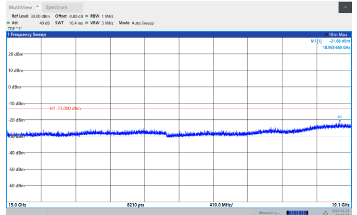
Band2-5MHz-QPSK-18900-1RB#0- Range:15000MHz~19100MHz
