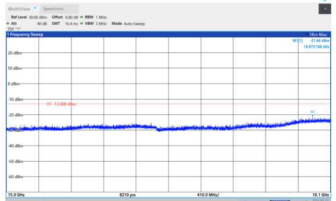
Band2-5MHz-QPSK-19175-1RB#0- Range:15000MHz~19100MHz
