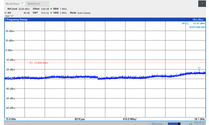
Band2-3MHz-QPSK-18900-1RB#0- Range:15000MHz~19100MHz
