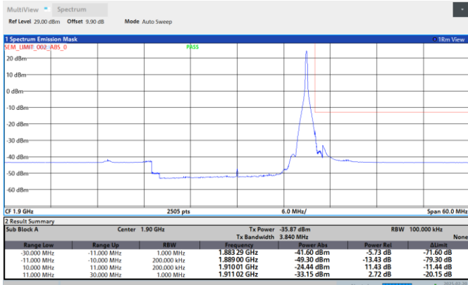
Band2-20MHz-16QAM-18700-1RB#0
