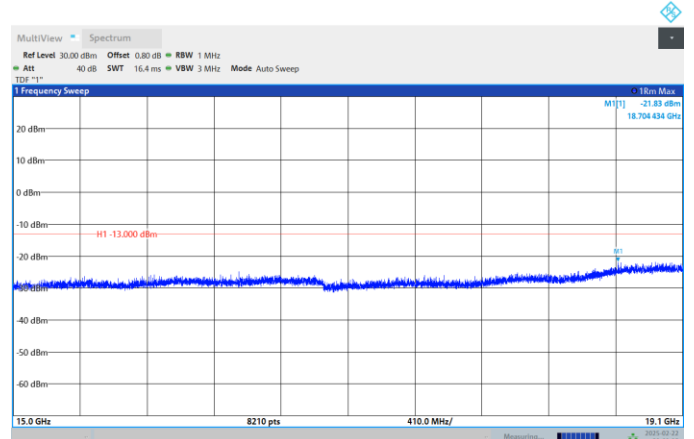
Band2-3MHz-QPSK-18615-1RB#0- Range:15000MHz~19100MHz
