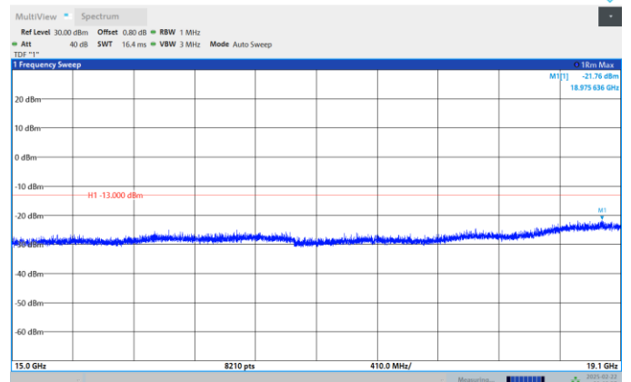
Band2-1.4MHz-QPSK-19193-1RB#0- Range:15000MHz~19100MHz
