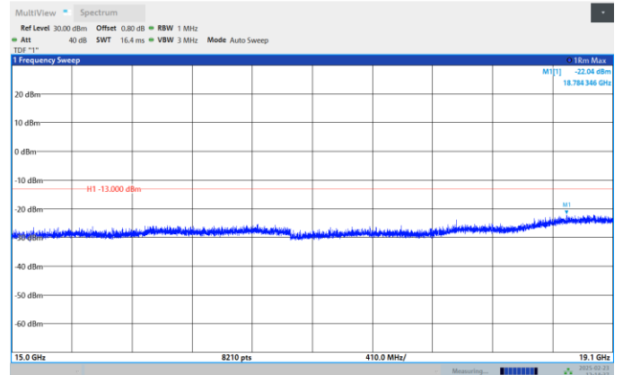
Band2-1.4MHz-QPSK-18900-1RB#0- Range:15000MHz~19100MHz
