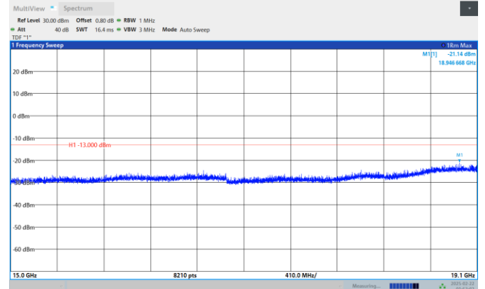
Band2-20MHz-QPSK-18900-1RB#0- Range:15000MHz~19100MHz
