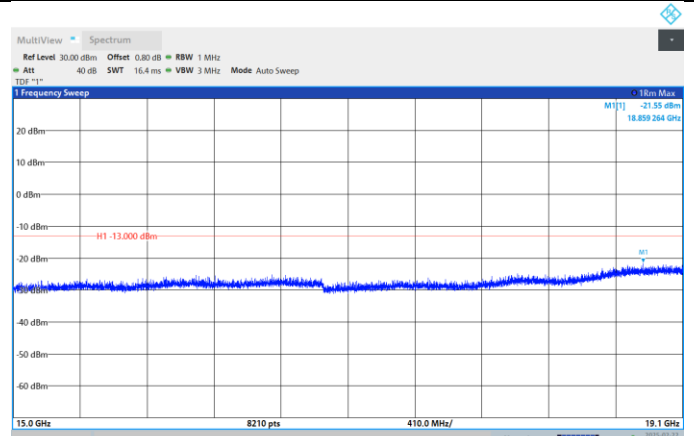
Band2-20MHz-QPSK-18700-1RB#0- Range:15000MHz~19100MHz
