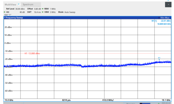
Band2-20MHz-QPSK-19100-1RB#0- Range:15000MHz~19100MHz
