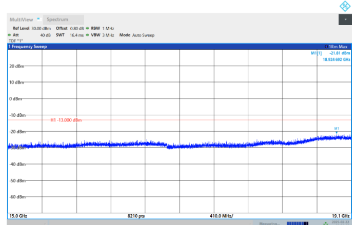
Band2-20MHz-QPSK-19100-1RB#0- Range:15000MHz~19100MHz
