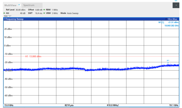
Band2-15MHz-QPSK-19125-1RB#0- Range:15000MHz~19100MHz
