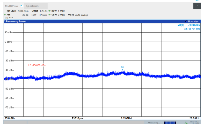
Band41-20MHz-QPSK-41490-1RB#0- Range:15000~26900MHz
