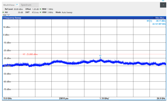
Band41-20MHz-QPSK-39750-1RB#0- Range:15000~26900MHz
