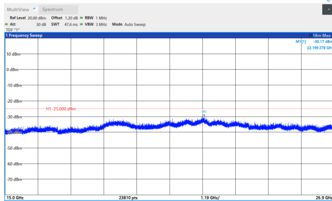
Band41-5MHz-QPSK-41565-1RB#0- Range:15000~26900MHz
