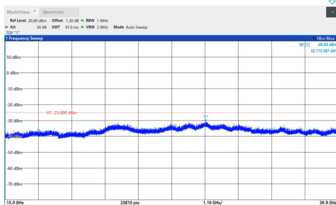
Band41-10MHz-QPSK-39700-1RB#0- Range:15000~26900MHz
