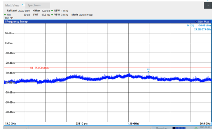
Band41-20MHz-QPSK-41490-1RB#0- Range:15000~26900MHz
