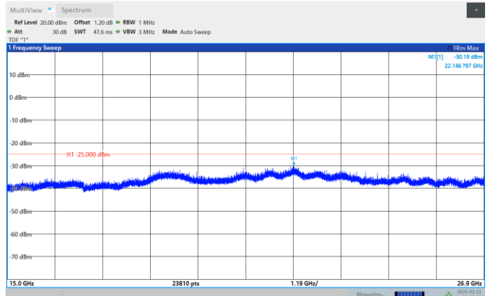
Band41-10MHz-QPSK-41540-1RB#0- Range:15000~26900MHz
