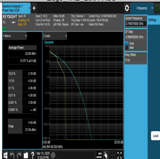
NTNV-N77-3700-3980-PC2-30-90-L-DFT-QPSK-Edge 1RB Left-PASS
