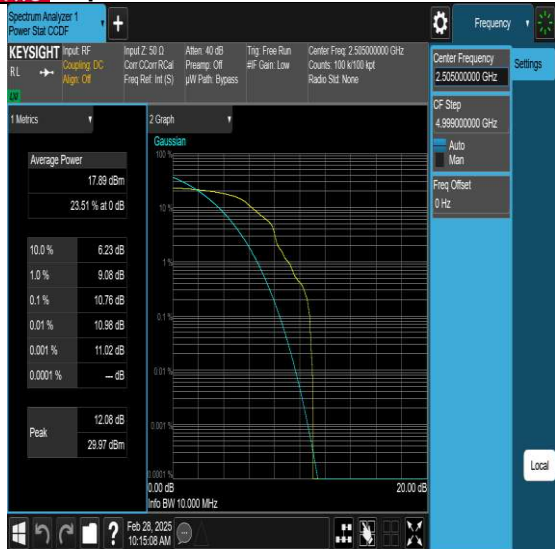
NTNV-N7-PC3-15-10-L-DFT-QPSK-Edge 1RB Left-PASS
