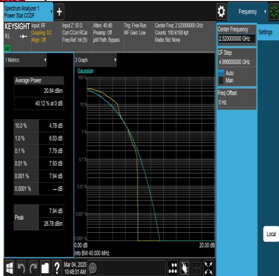
NTV-N7-PC3-15-40-L-DFT-QPSK-Edge 1RB Left-PASS
