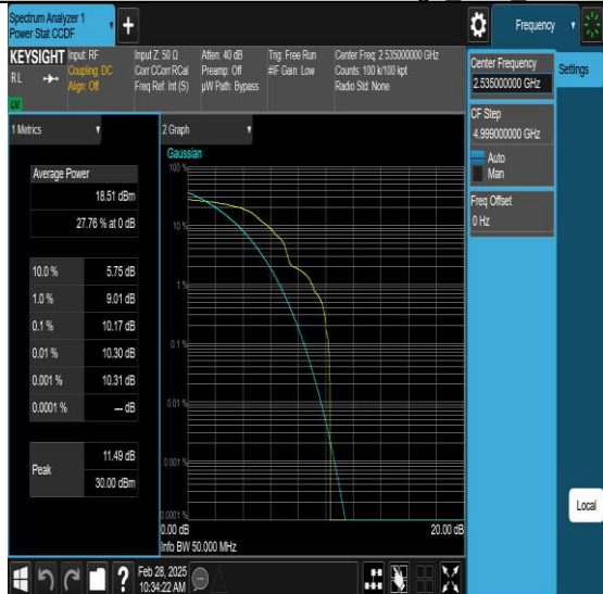
NTNV-N7-PC3-15-50-M-DFT-QPSK-Edge 1RB Left-PASS
