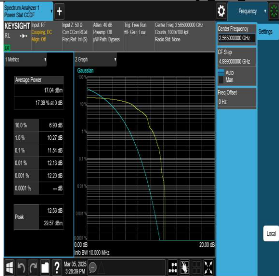
NTNV-N7-PC3-15-10-H-DFT-QPSK-Edge 1RB Left-PASS
