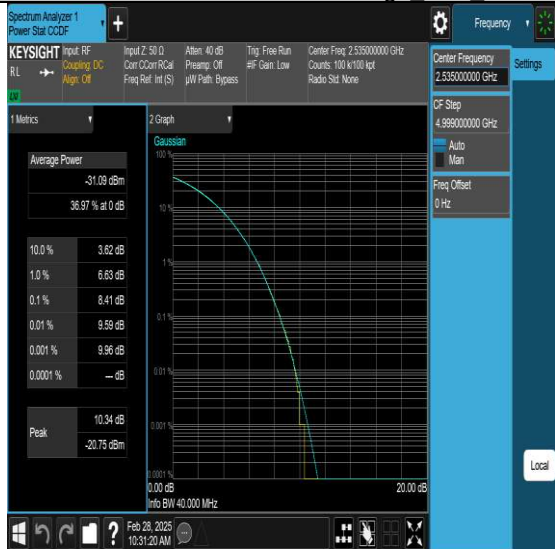
NTV-N7-PC3-15-40-M-DFT-QPSK-Edge 1RB Left-PASS
