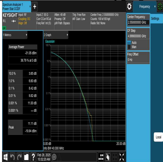
NTV-N7-PC3-15-40-H-DFT-QPSK-Edge 1RB Left-PASS
