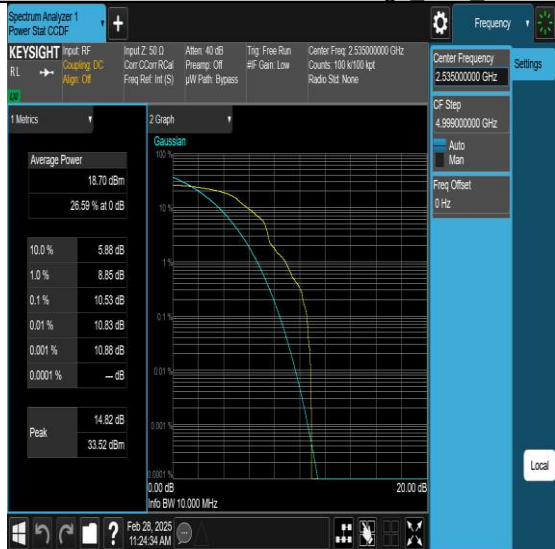
NTNV-N7-PC3-15-10-M-DFT-QPSK-Edge 1RB Left-PASS
