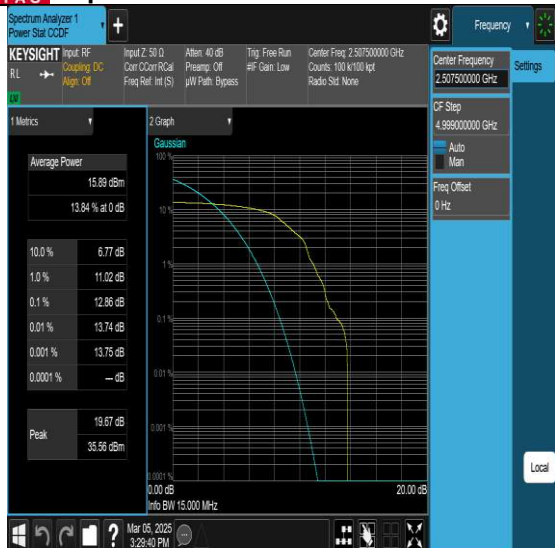
NTNV-N7-PC3-15-15-L-DFT-QPSK-Edge 1RB Left-PASS
