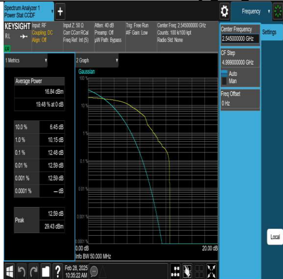
NTNV-N7-PC3-15-50-H-DFT-QPSK-Edge 1RB Left-PASS
