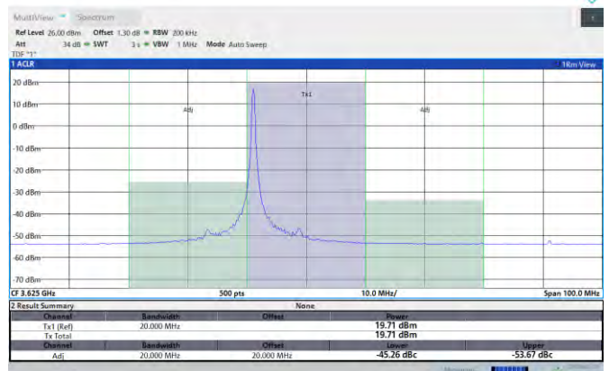
Band48-20MHz-QPSK-55990-1RB#99-PASS
