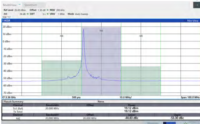
Band48-20MHz-QPSK-55340-1RB#99-PASS
