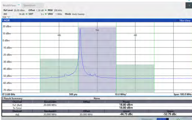
Band48-20MHz-QPSK-56640-1RB#99-PASS
