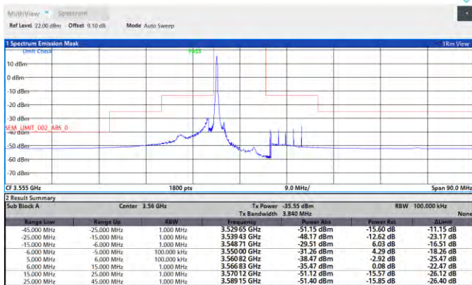
Band48-10MHz-QPSK-55290-50RB#0-PASS
