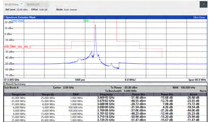
Band48-10MHz-QPSK-56690-1RB#49-PASS
