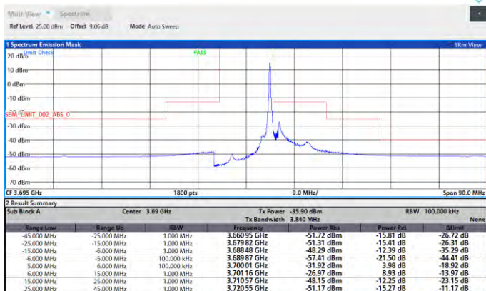
Band48-10MHz-QPSK-56690-50RB#0-PASS
