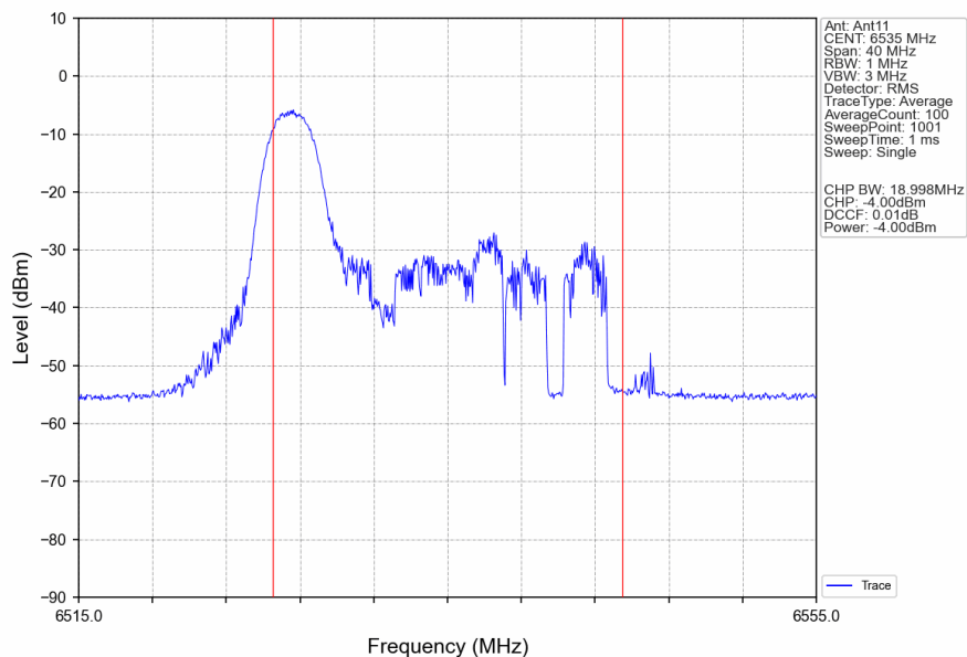
802.11ax(HEW20)_LCH_6535MHz_RU26_Left_Ant11_NTNV
