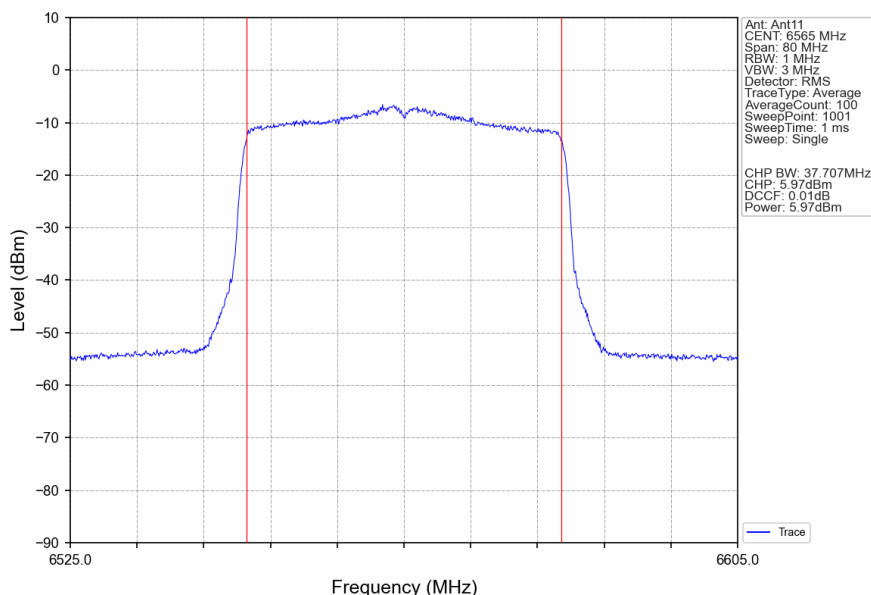
802.11ax(HEW40)_LCH_6565MHz_RU484_Left_Ant11_NTNV
