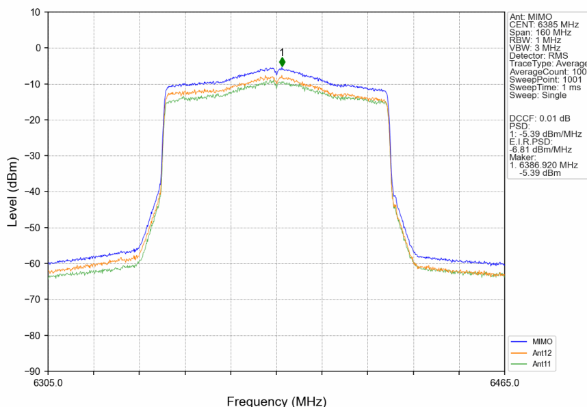
802.11ax(HEW80)_HCH_6385MHz_RU996_Left_MIMO_NTNV
