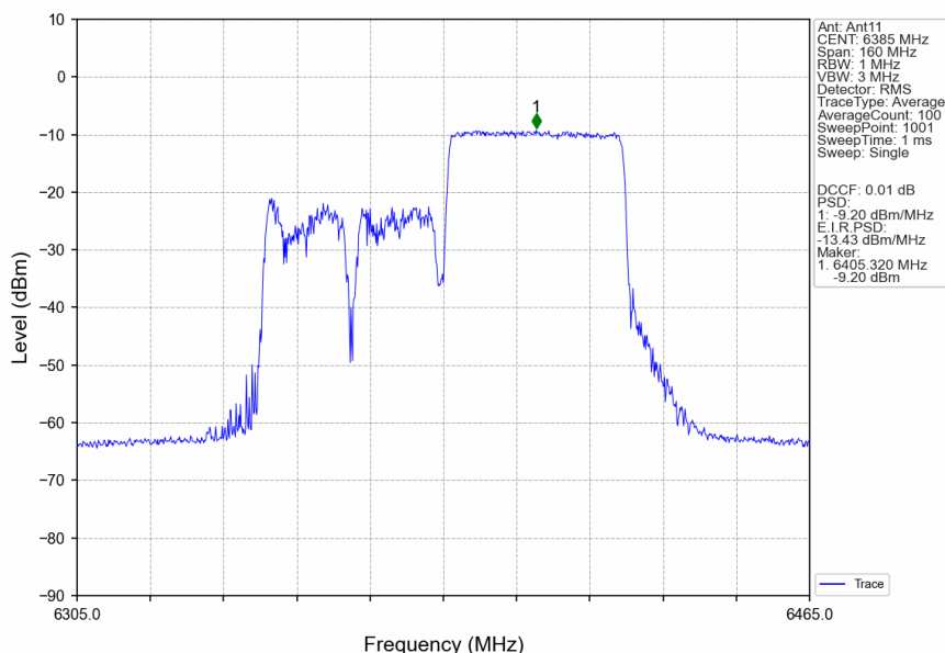
802.11ax(HEW80)_HCH_6385MHz_RU484_Right_Ant11_NTNV
