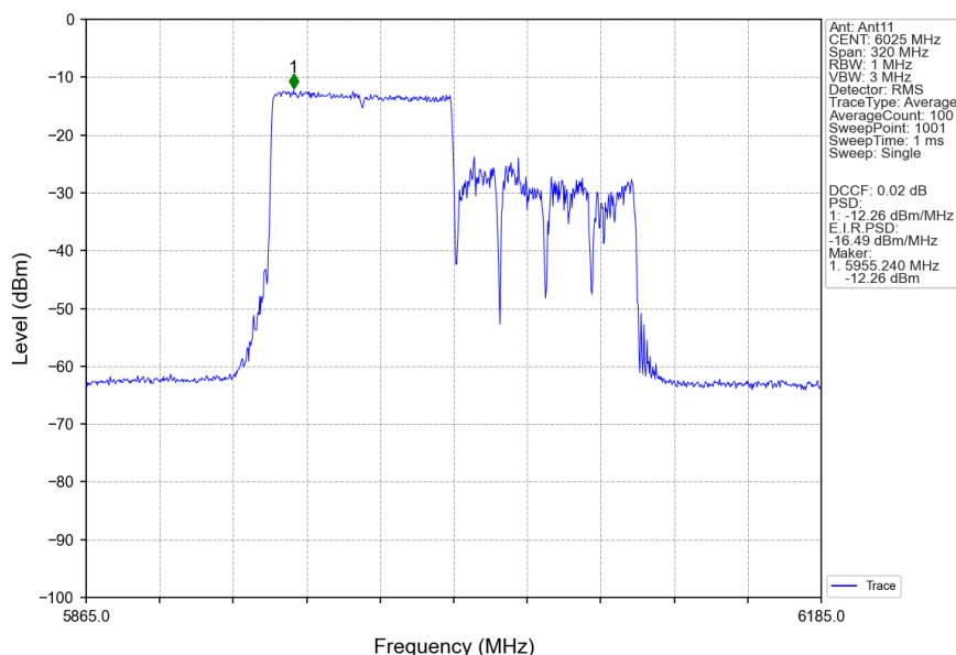
802.11ax(HEW160)_LCH_6025MHz_RU996_Left_Ant11_NTNV
