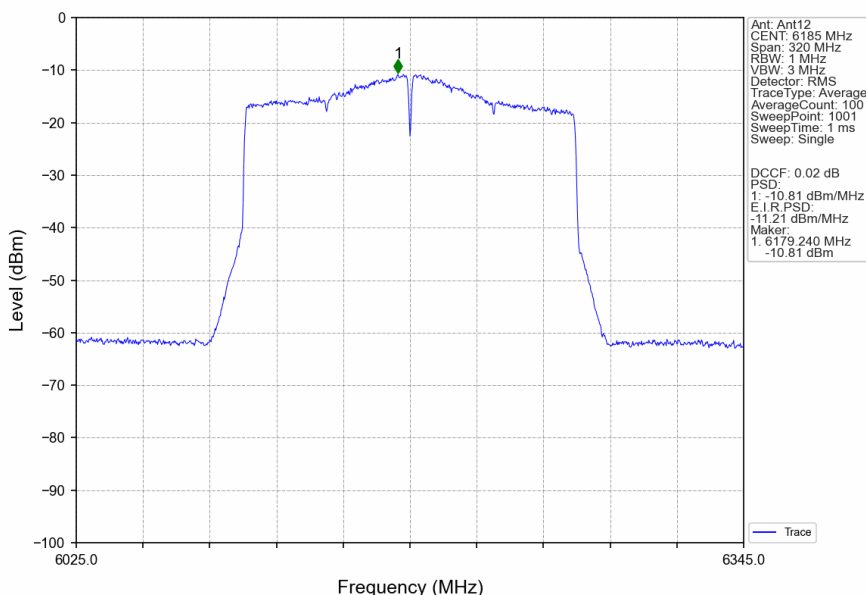
802.11ax(HEW160)_MCH_6185MHz_2xRU996_Left_Ant12_NTNV
