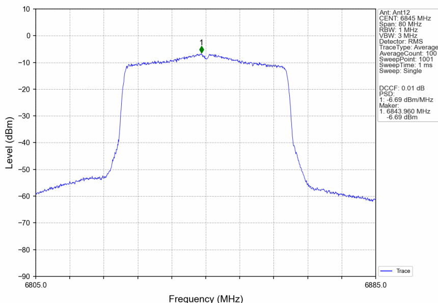
802.11ax(HEW40)_HCH_6845MHz_RU484_Left_Ant12_NTNV
