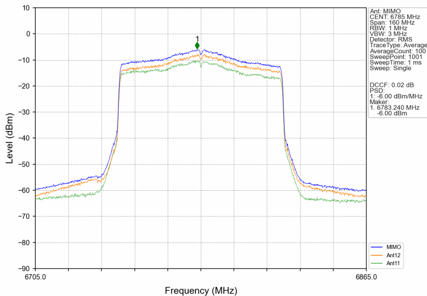
802.11ax(HEW80)_HCH_6785MHz_RU996_Left_MIMO_NTNV
