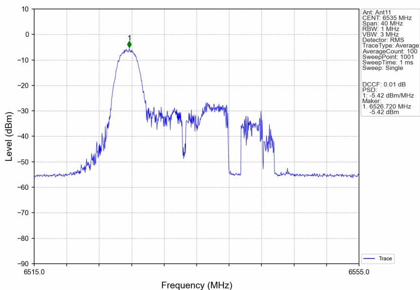
802.11ax(HEW20)_LCH_6535MHz_RU26_Left_Ant11_NTNV
