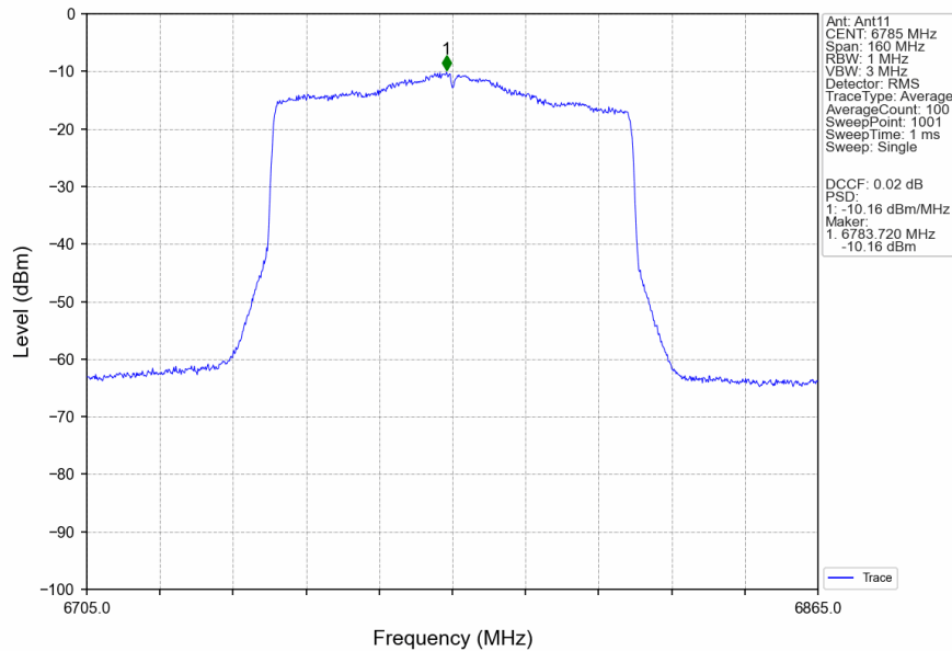
802.11ax(HEW80)_HCH_6785MHz_RU996_Left_MIMO_NTNV
