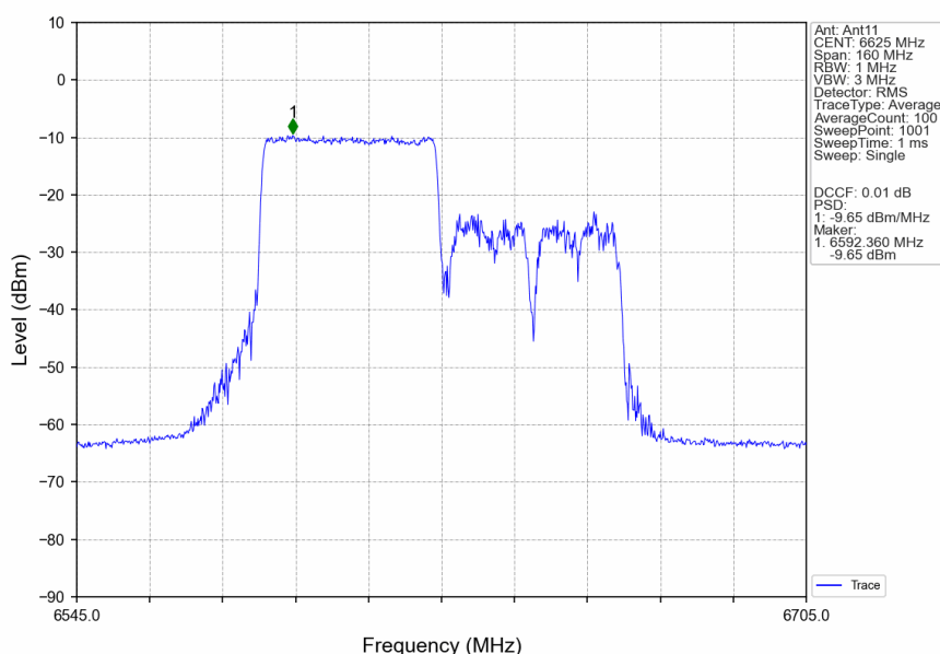
802.11ax(HEW80)_LCH_6625MHz_RU484_Left_Ant11_NTNV
