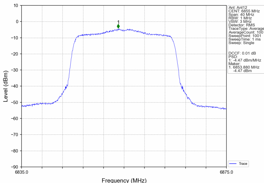
802.11ax(HEW20)_HCH_6855MHz_RU242_Left_Ant12_NTNV
