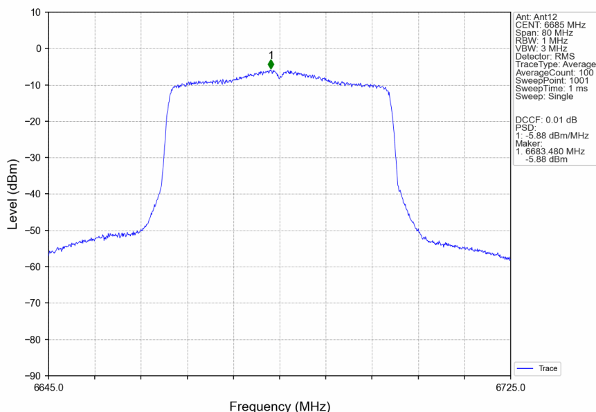
802.11ax(HEW40)_MCH_6685MHz_RU484_Left_Ant12_NTNV
