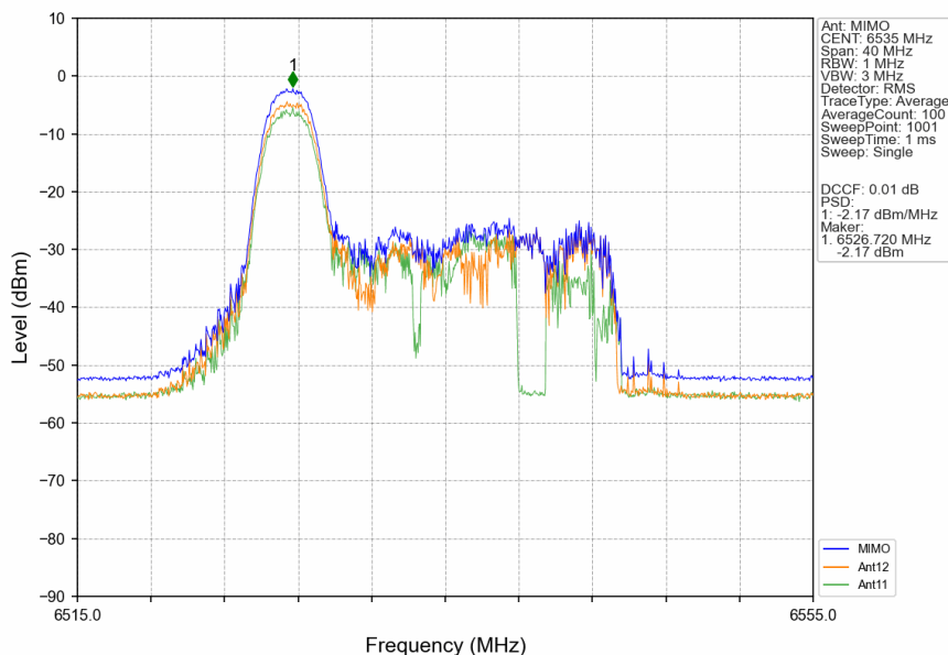
802.11ax(HEW20)_LCH_6535MHz_RU52_Left_Ant12_NTNV
