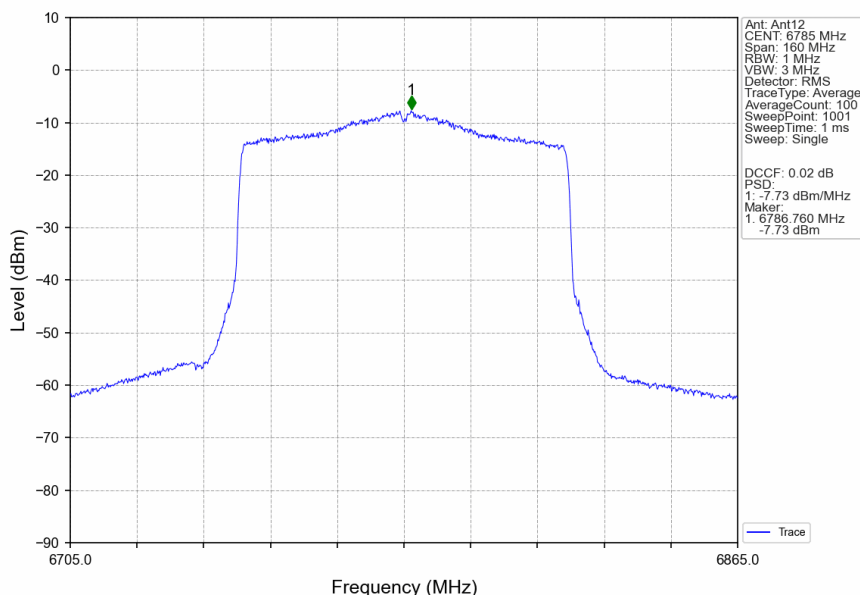
802.11ax(HEW80)_HCH_6785MHz_RU996_Left_Ant12_NTNV
