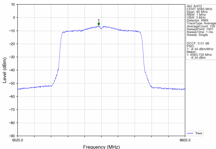
802.11ax(HEW40)_LCH_6565MHz_RU484_Left_Ant12_NTNV
