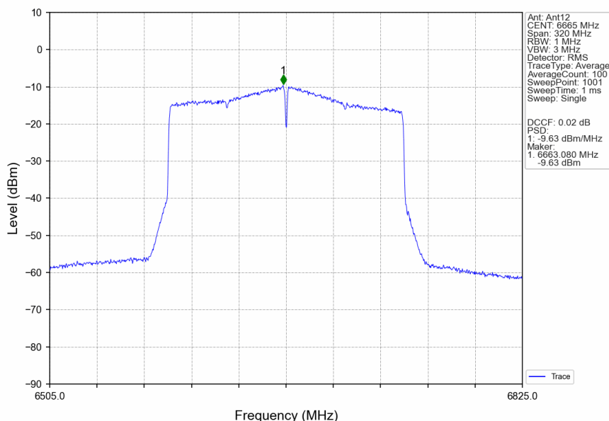
802.11ax(HEW160)_MCH_6665MHz_2xRU996_Left_Ant12_NTNV
