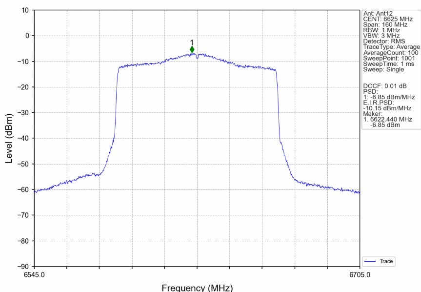
802.11ax(HEW80)_LCH_6625MHz_RU996_Left_Ant12_NTNV
