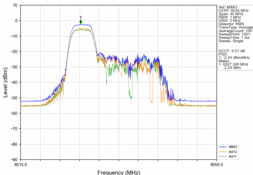
802.11ax(HEW20) LCH 6535MHz RU52 Left MIMO NTNV
