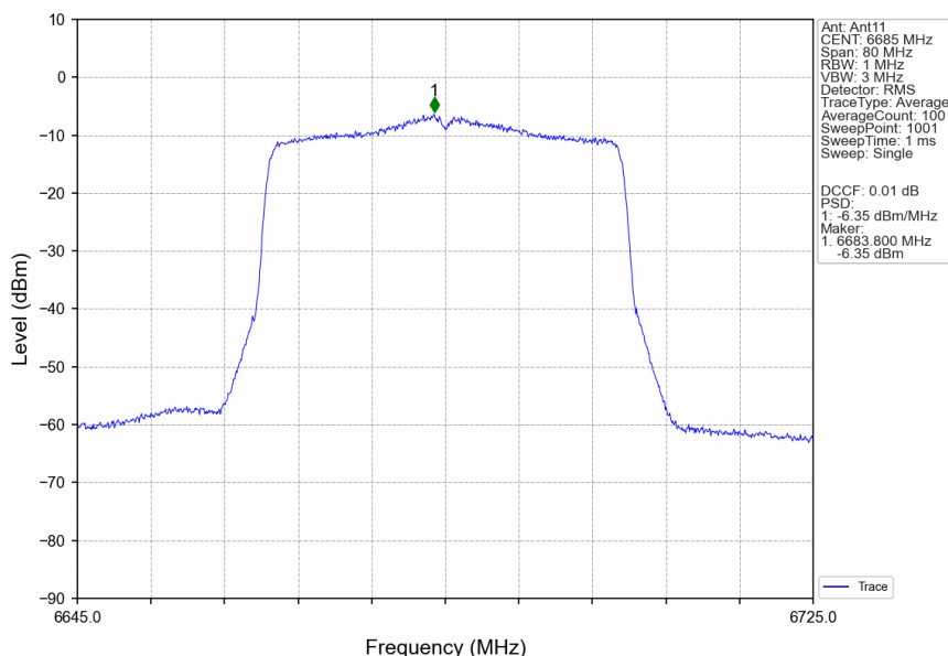
802.11ax(HEW40) MCH 6685MHz RU484 Left MIMO NTN
