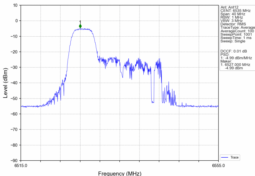
802.11ax(HEW20) LCH 6535MHz RU52 Left Ant12 NTN
