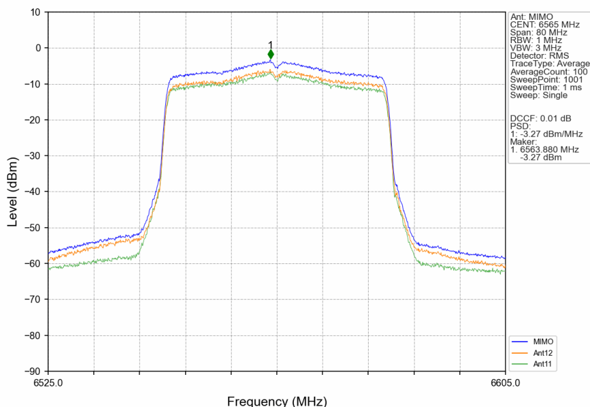
802.11ax(HEW40) LCH 6565MHz RU484 Left MIMO NTVN
