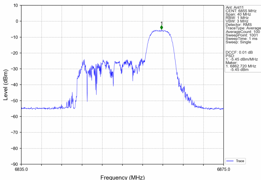
802.11ax(HEW20) HCH 6855MHz RU52 Right MIMO NTN
