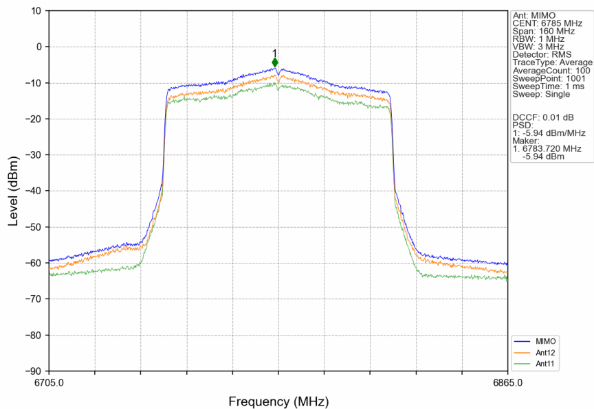
802.11ax(HEW80) HCH 6785MHz RU996 Left MIMO NTN
