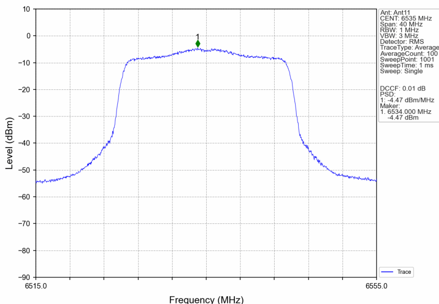
802.11ax(HEW20) LCH 6535MHz RU242 Left MIMO NTN
