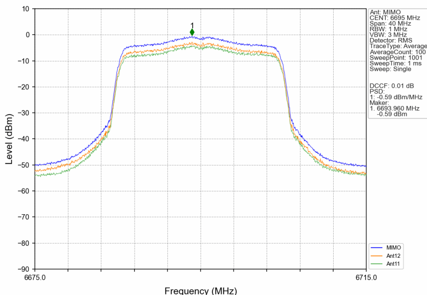
802.11ax(HEW20) MCH 6695MHz RU242 Left MIMO NTN
