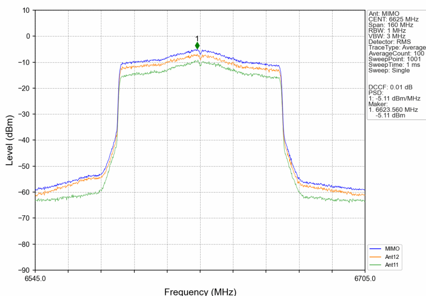
802.11ax(HEW80) LCH 6625MHz RU996 Left MIMO NTN
