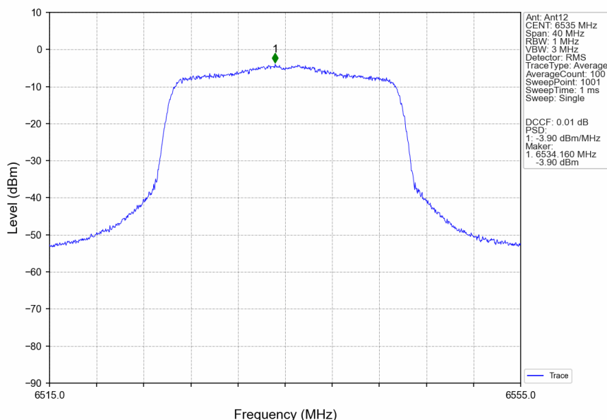
802.11ax(HEW20) LCH 6535MHz RU242 Left Ant12 NTN
