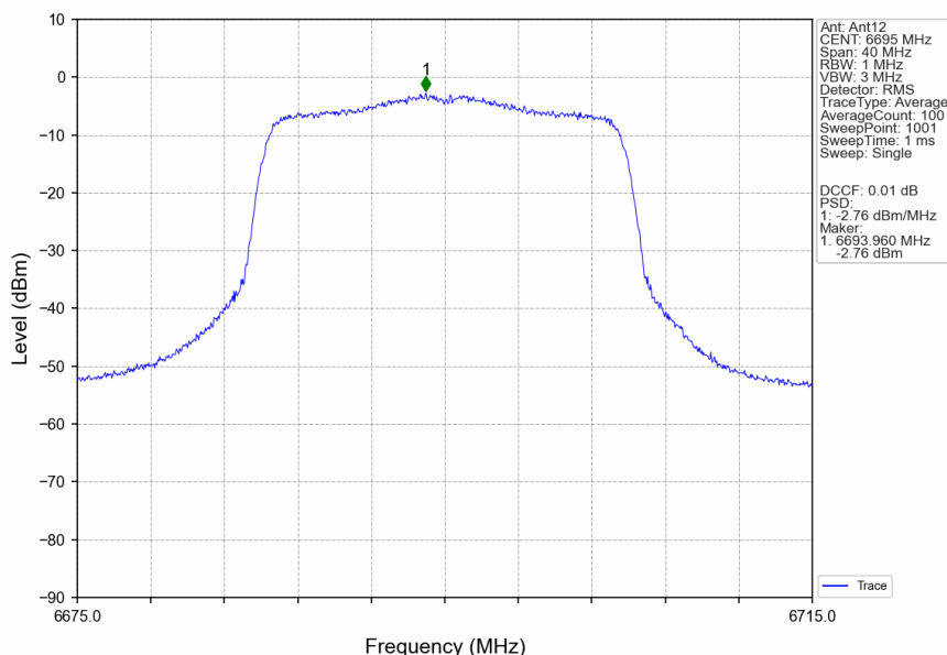
802.11ax(HEW20) MCH_6695MHz RU242 Left Ant12 NTN
