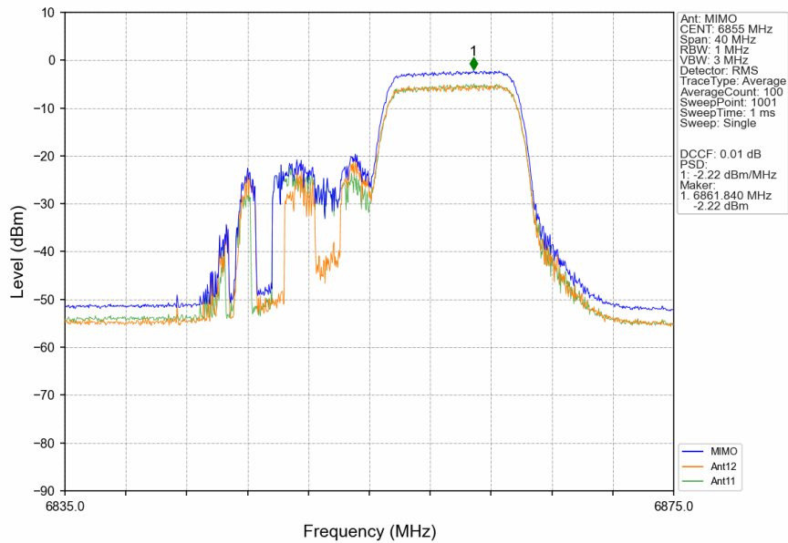
802.11ax(HEW20) HCH 6855MHz RU242 Left Ant12 NTN
