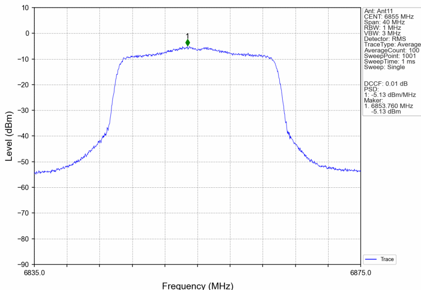
802.11ax(HEW20) HCH 6855MHz RU242 Left MIMO NTN
