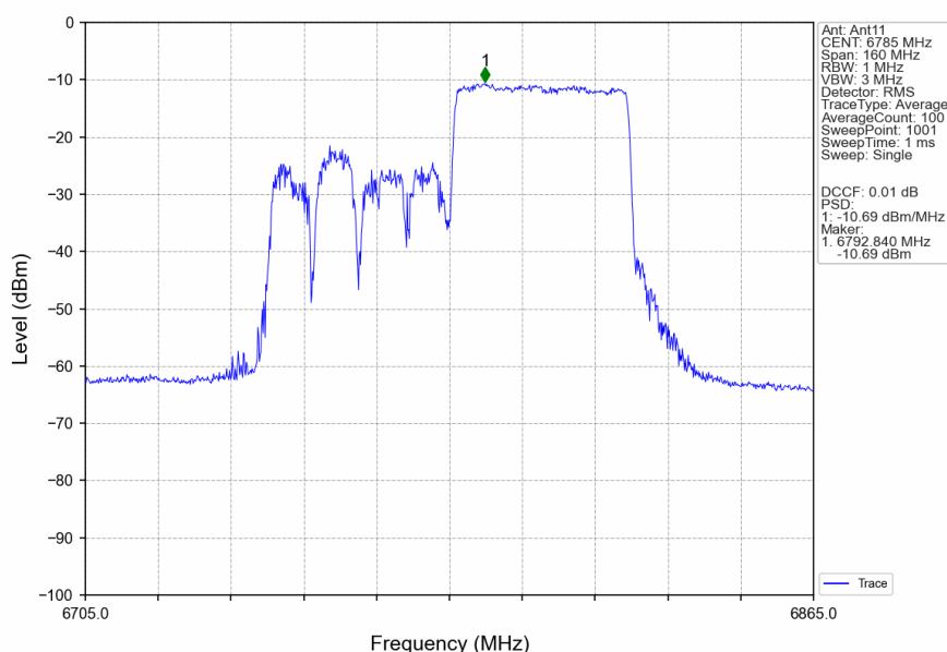
802.11ax(HEW80) HCH 6785MHz RU484 Right Ant11 NTNV
