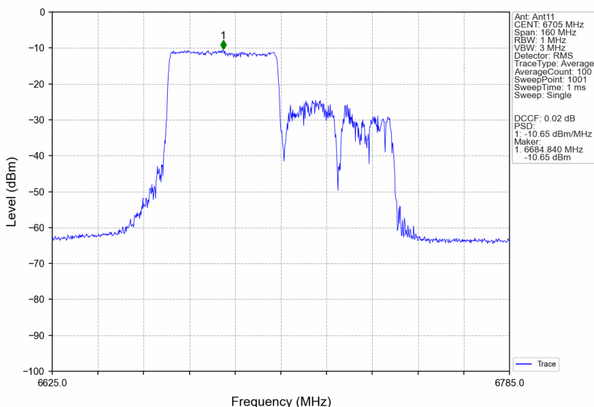
802.11ax(HEW80) MCH 6705MHz RU484 Left Ant11 NTN
