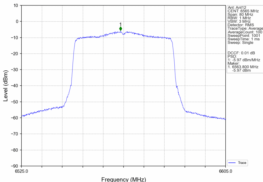
802.11ax(HEW40) LCH 6565MHz RU484 Left Ant12 NTN
