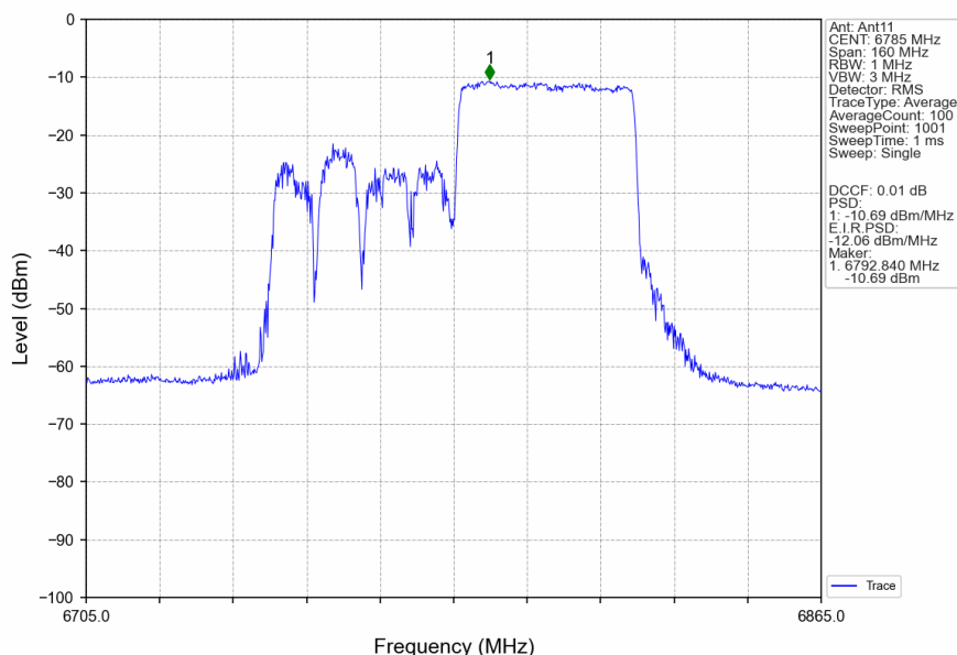
802.11ax(HEW80) HCH 6785MHz RU484 Right Ant11 NTN
