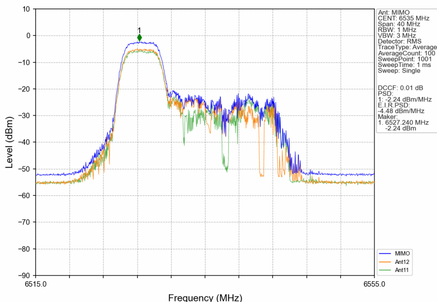
802.11ax(HEW20) LCH 6535MHz RU52 Left MIMO NTVN
