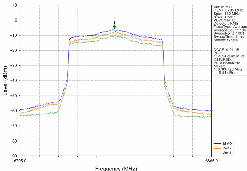
802.11ax(HEW80) HCH 6785MHz RU996 Left MIMO NTN
