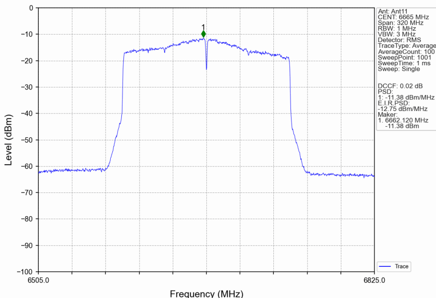
802.11ax(HEW160) MCH 6665MHz 2xRU996 Left MIMO NTVN
