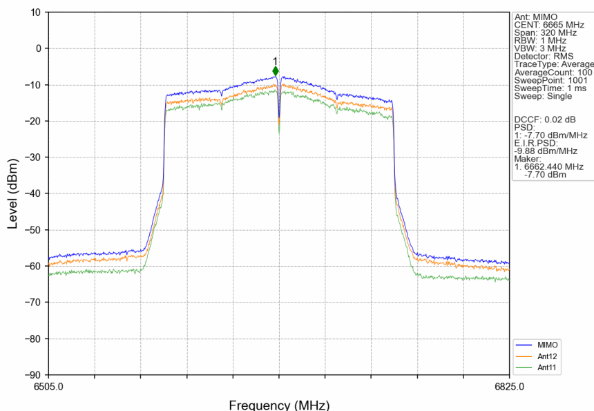
802.11ax(HEW160) MCH 6665MHz 2xRU996 Left MIMO NTVN
