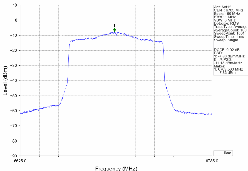
802.11ax(HEW80) MCH 6705MHz RU996 Left Ant12 NTN
