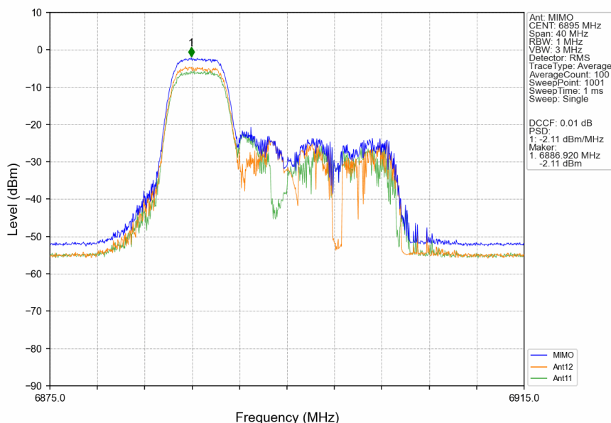
802.11ax(HEW20) LCH 6895MHz RU52 Left MIMO NTVN
