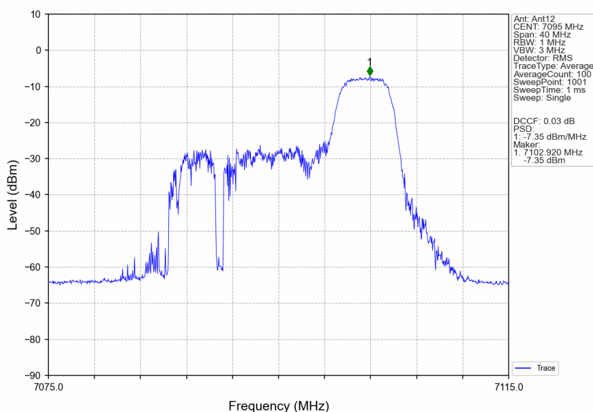
802.11ax(HEW20) HCH_7095MHz_RU52_Right_Ant12_NTNV
