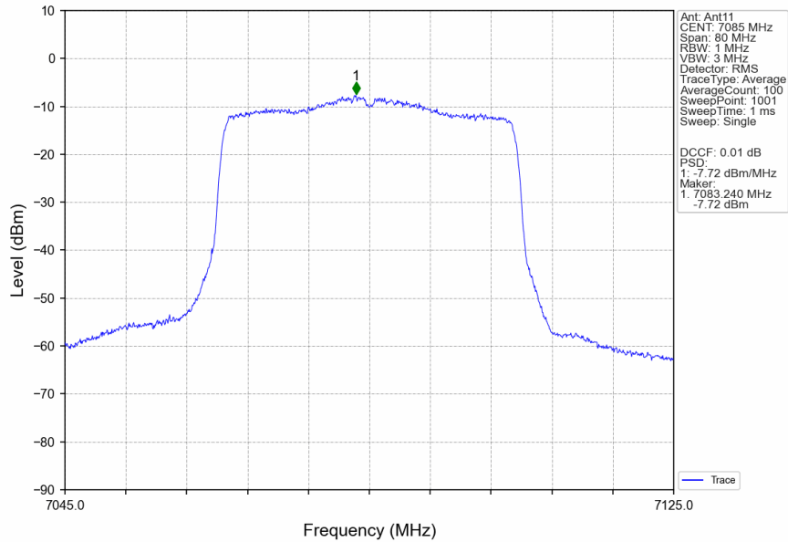
802.11ax(HEW40) HCH 7085MHz RU484 Left MIMO NTN
