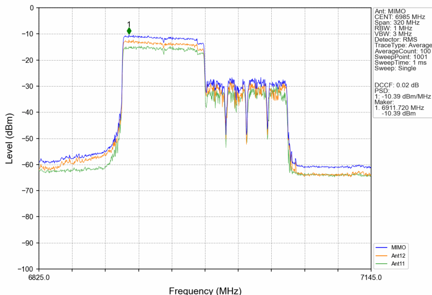
802.11ax(HEW160) MCH 6985MHz 2xRU996 Left Ant12 NTNv
