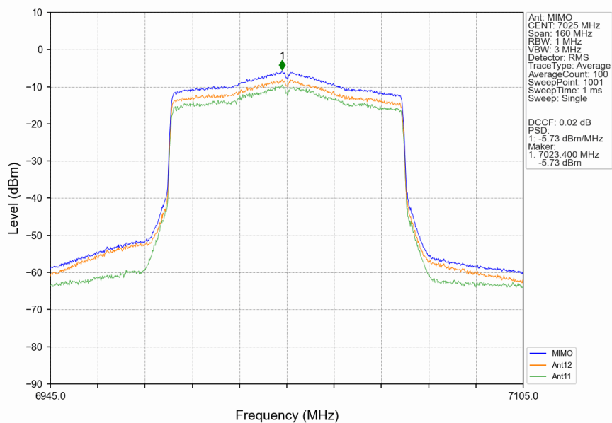
802.11ax(HEW80) HCH 7025MHz RU996 Left MIMO NTN
