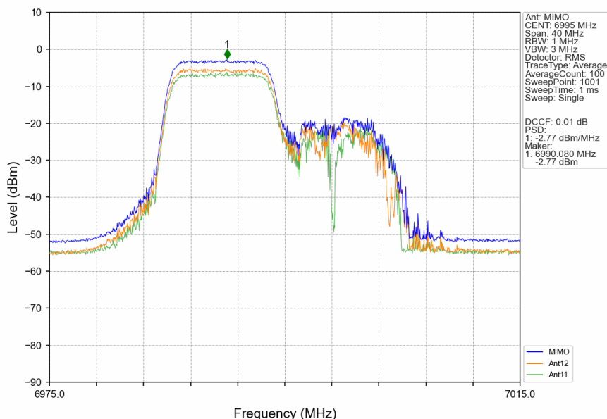
802.11ax(HEW20) MCH_6995MHz RU242 Left Ant12 NTN
