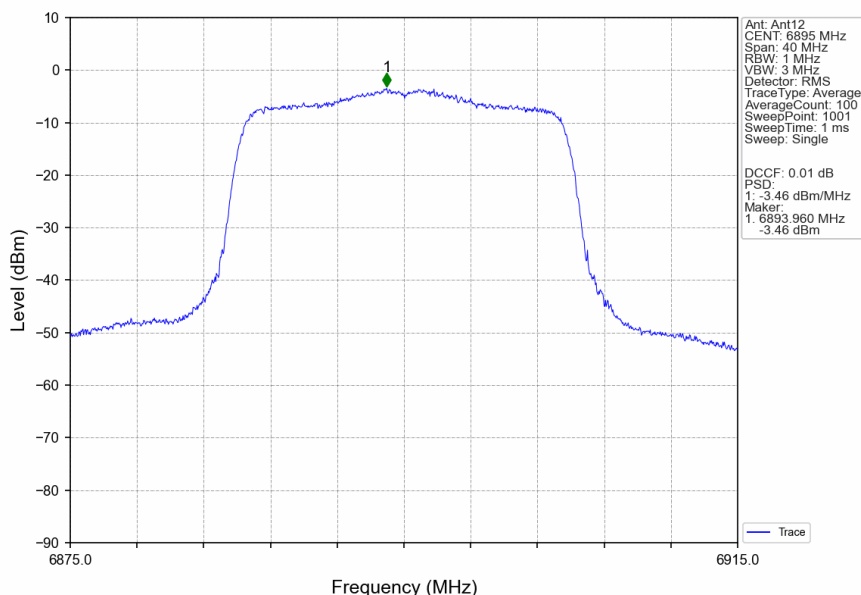
802.11ax(HEW20) LCH 6895MHz RU242 Left Ant12 NTN
