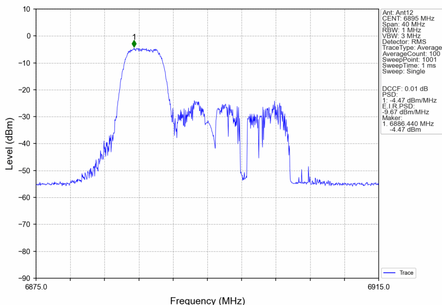
802.11ax(HEW20) LCH 6895MHz RU52 Left Ant12 NTN
