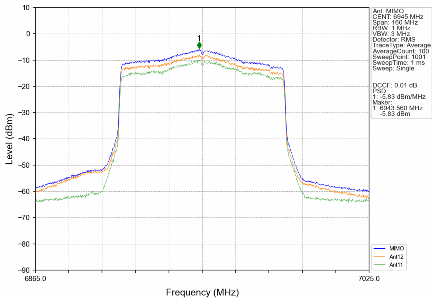
802.11ax(HEW80) LCH 6945MHz RU996 Left MIMO NTN
