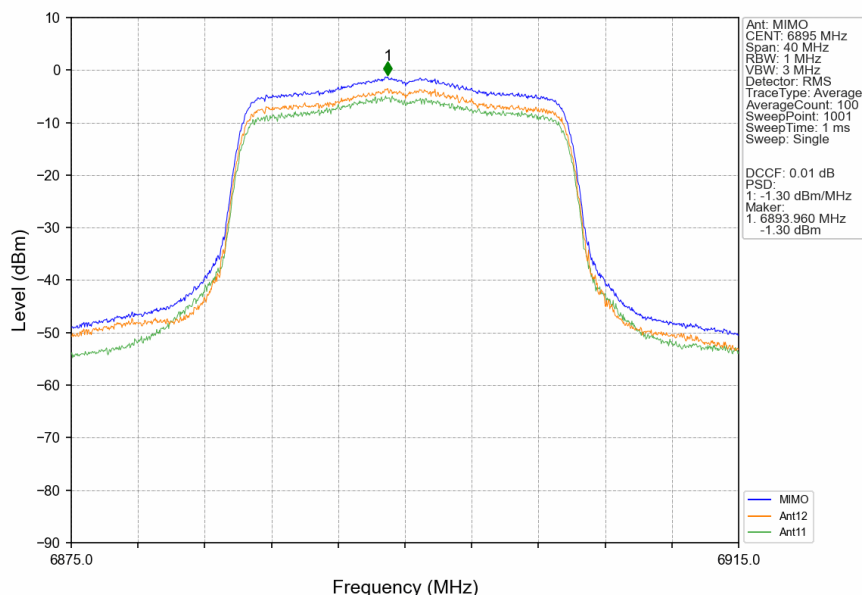
802.11ax(HEW20) LCH 6895MHz RU242 Left MIMO NTN
