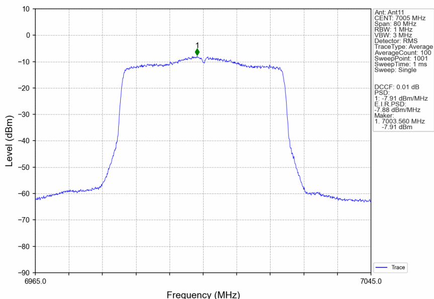
802.11ax(HEW40) MCH 7005MHz RU484 Left MIMO NTN
