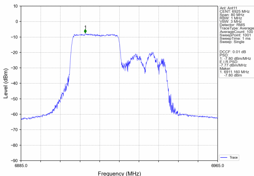
802.11ax(HEW40) LCH 6925MHz RU242 Left Ant11 NTNV
