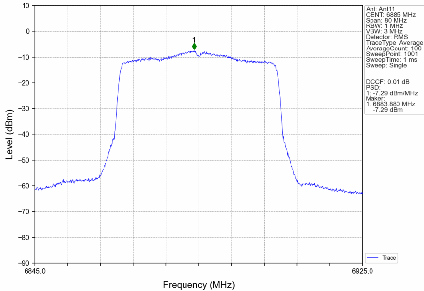
802.11ax(HEW40) HCH 6885MHz RU484 Left MIMO NTN
