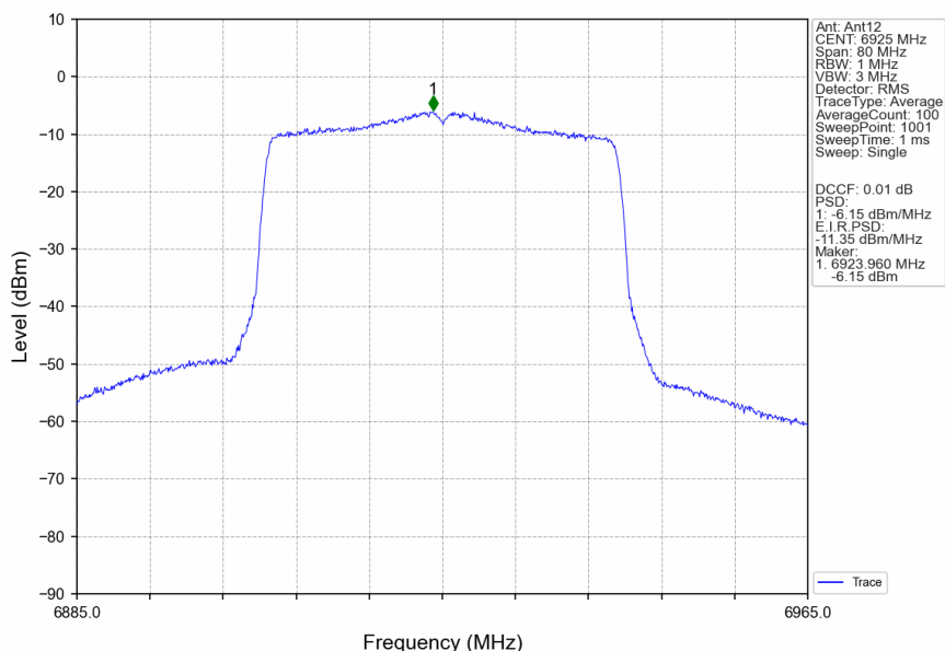
802.11ax(HEW40) LCH 6925MHz RU484 Left Ant12 NTN
