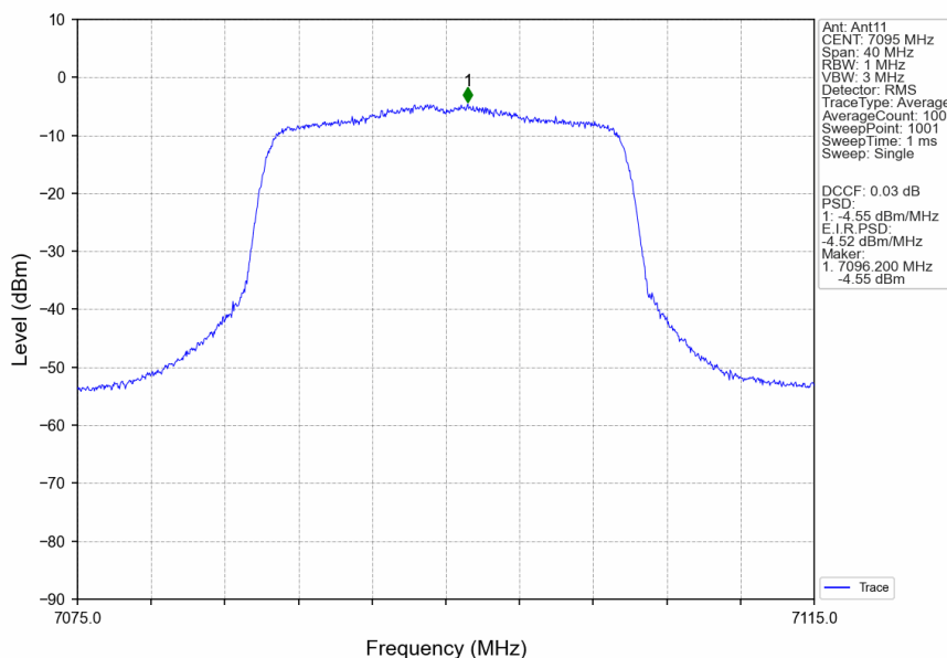
802.11ax(HEW20) HCH 7095MHz RU242 Left MIMO NTN
