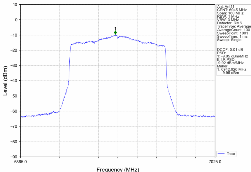
802.11ax(HEW80) LCH 6945MHz RU996 Left MIMO NTN
