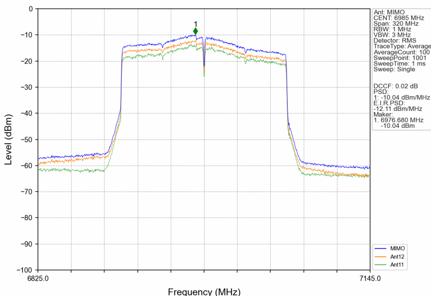
802.11ax(HEW160) MCH 6985MHz 2xRU996 Left MIMO NTNV
