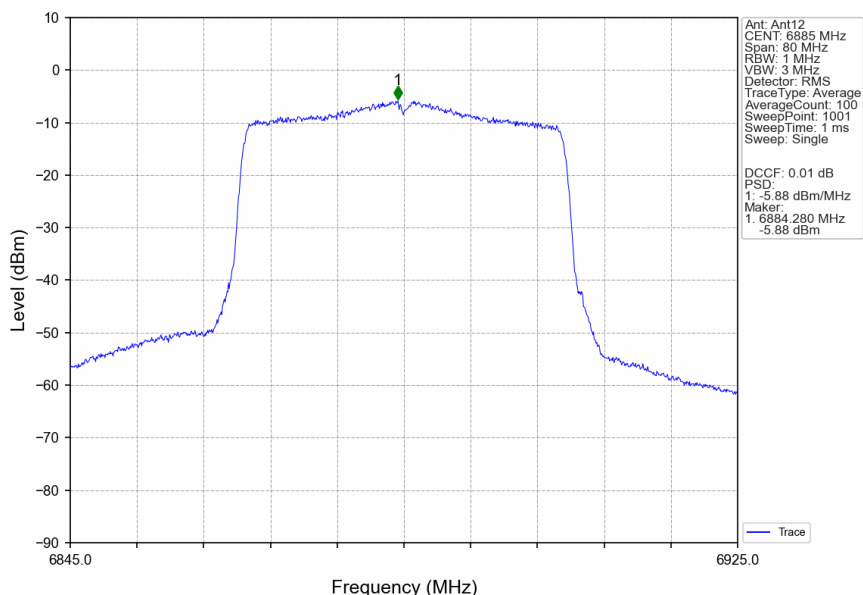
802.11ax(HEW40) HCH 6885MHz RU484 Left Ant12 NTN
