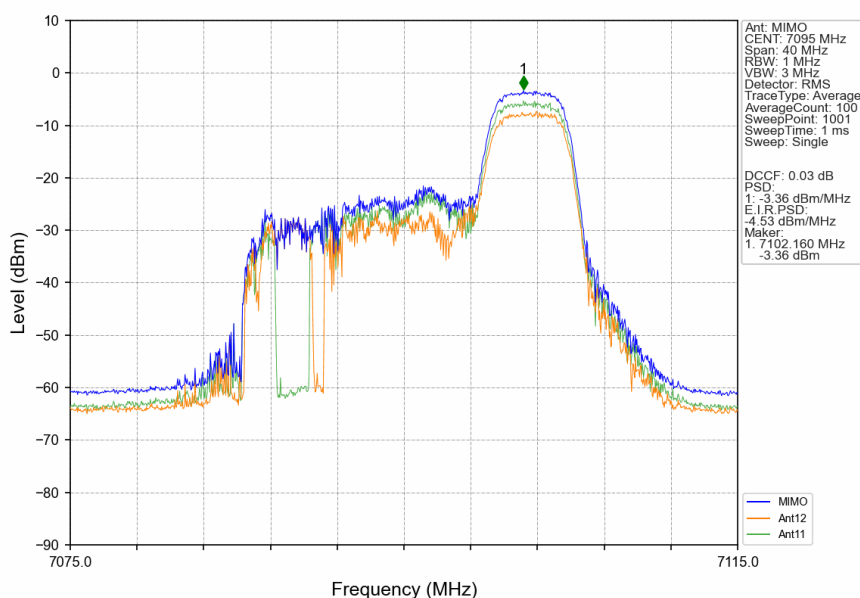
802.11ax(HEW20) HCH 7095MHz RU52 Right MIMO NTN
