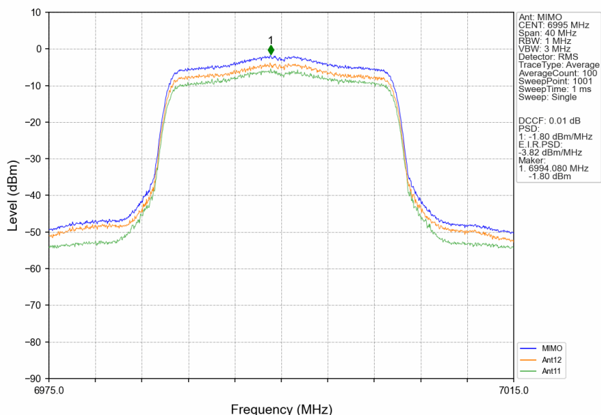
802.11ax(HEW20) MCH 6995MHz RU242 Left MIMO NTN
