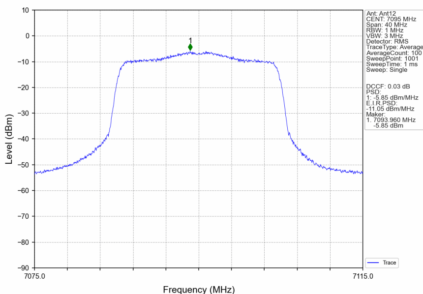
802.11ax(HEW20)_HCH_7095MHz_RU242_Left_Ant12_NTNV
