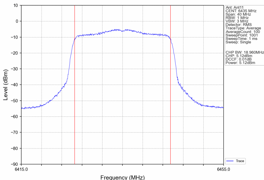
802.11ax(HEW20) LCH 6435MHz RU242 Left Ant11 NTNV
