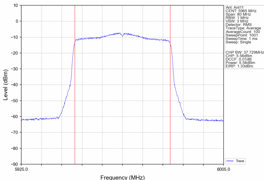
802.11ax(HEW40) LCH 5965MHz RU484 Left Ant11 NTN
