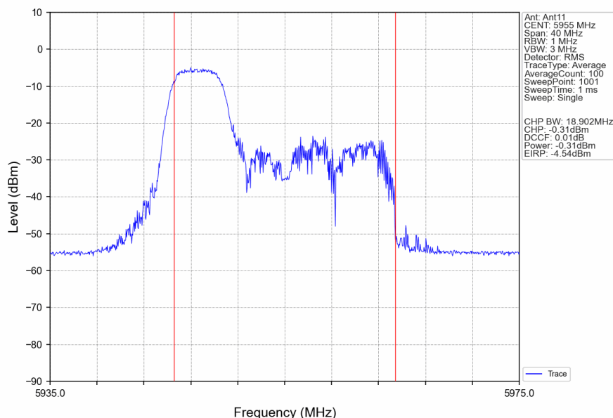
802.11ax(HEW20) LCH 5955MHz RU52 Left Ant11 NTNV
