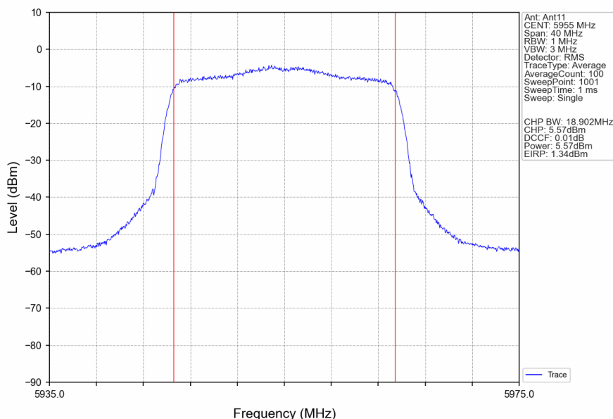
802.11ax(HEW20) LCH 5955MHz RU242 Left Ant11 NTN
