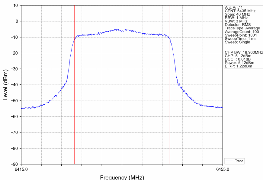
802.11ax(HEW20) LCH 6435MHz RU242 Left Ant11 NTN
