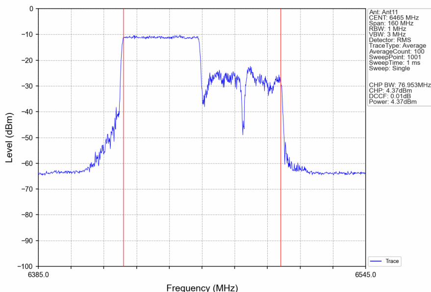
802.11ax(HEW80) LCH 6465MHz RU484 Left Ant11 NTNV
