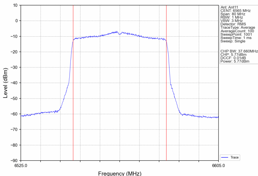
802.11ax(HEW40) LCH 6565MHz RU484 Left Ant11 NTN
