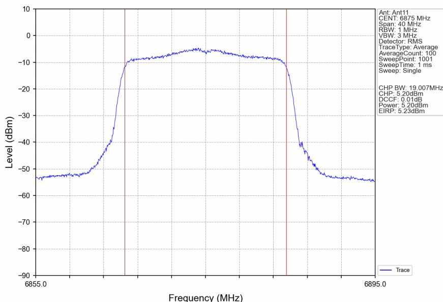
802.11ax(HEW20) HCH 6875MHz RU242 Left Ant11 NTN
