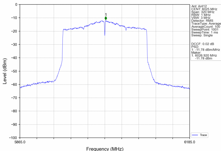
802.11ax(HEW160) LCH 6025MHz 2xRU996 Left Ant12 NTN
