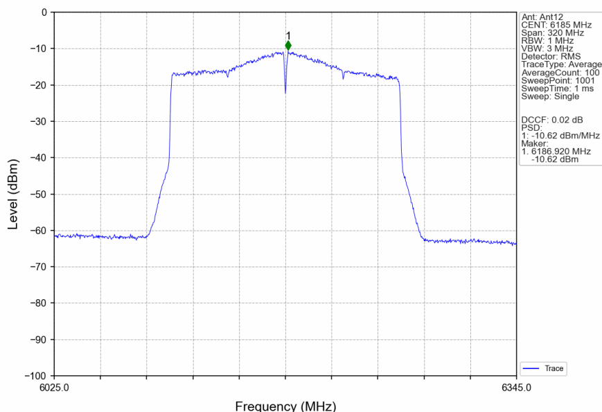
802.11ax(HEW160) MCH 6185MHz 2xRU996 Left Ant12 NTNv
