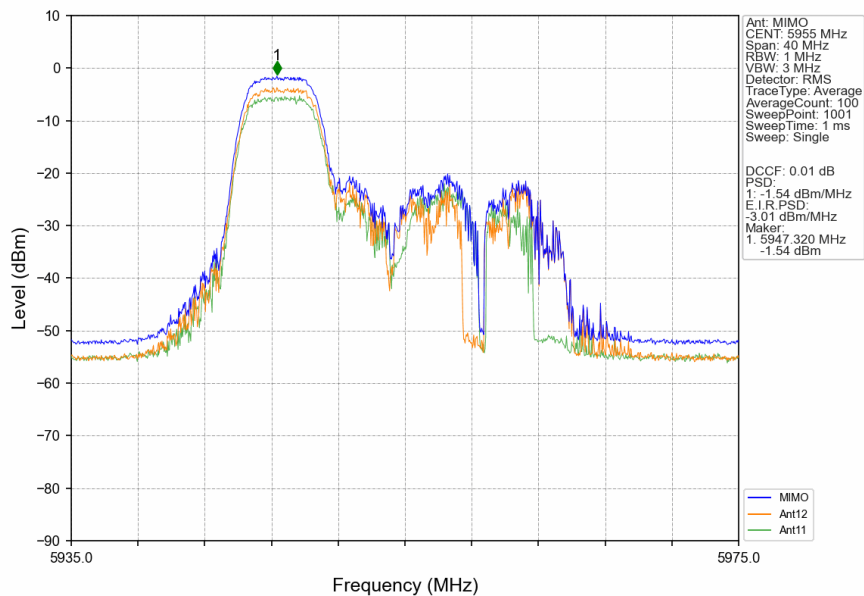
802.11ax(HEW20) LCH 5955MHz RU52 Left MIMO NTVN
