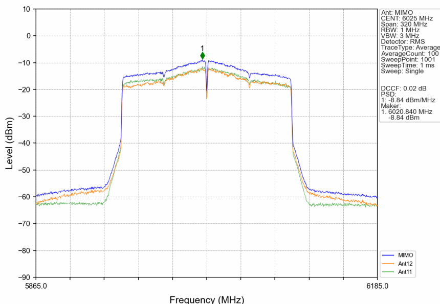
802.11ax(HEW160) LCH 6025MHz 2xRU996 Left MIMO NTNV
