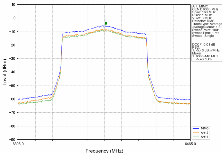
802.11ax(HEW80) HCH 6385MHz RU996 Left MIMO NTN
