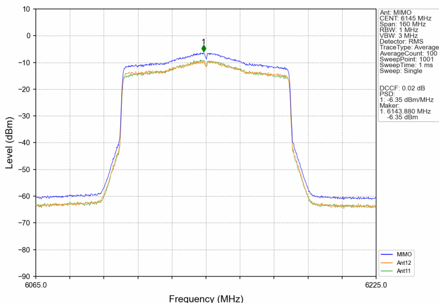
802.11ax(HEW80) MCH 6145MHz RU996 Left MIMO NTN
