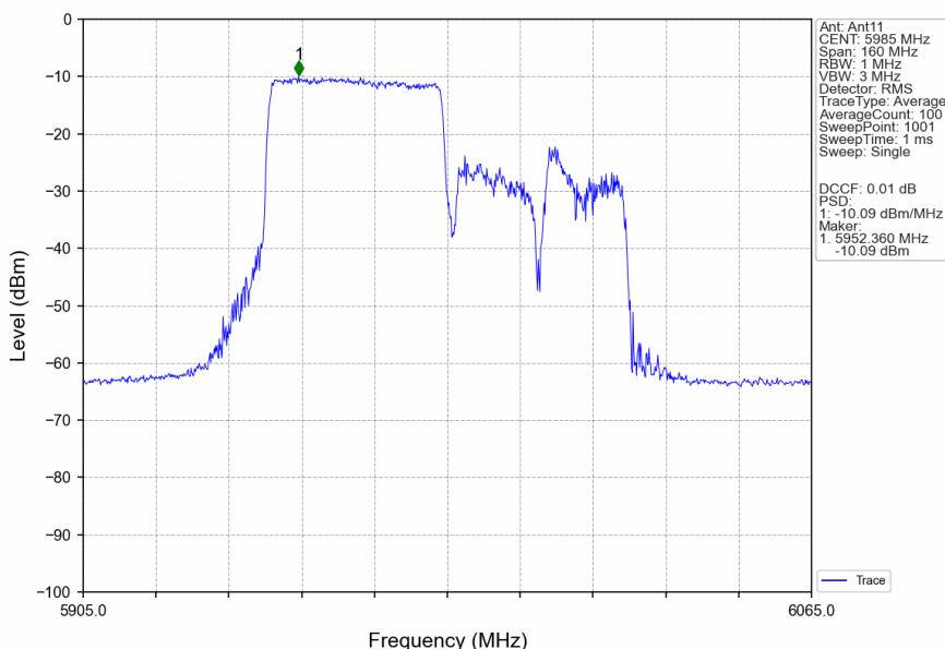
802.11ax(HEW80) LCH 5985MHz RU484 Left Ant11 NTN
