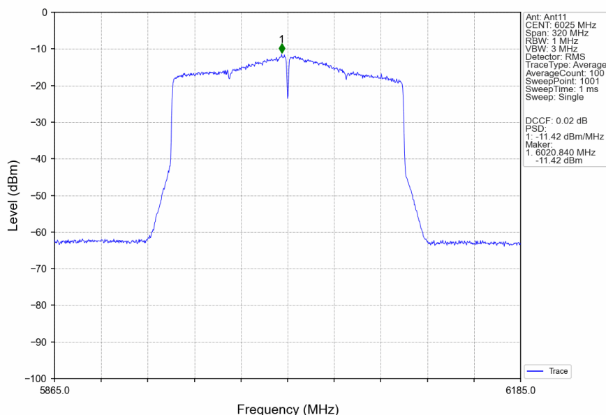
802.11ax(HEW160) LCH 6025MHz 2xRU996 Left MIMO NTNV
