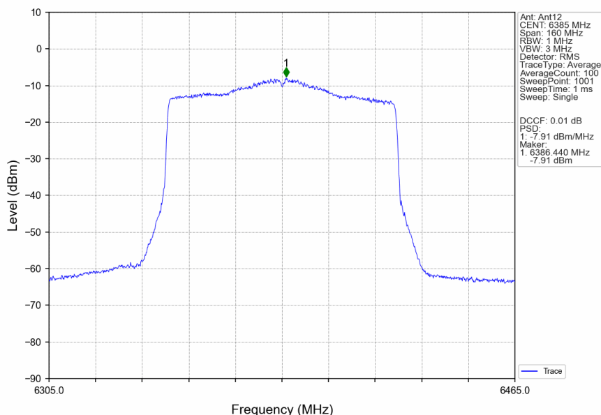
802.11ax(HEW80) HCH 6385MHz RU996 Left Ant12 NTN
