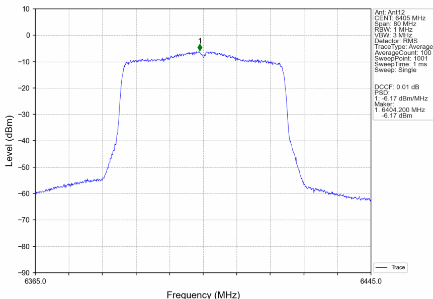
802.11ax(HEW40) HCH 6405MHz RU484 Left Ant12 NTN
