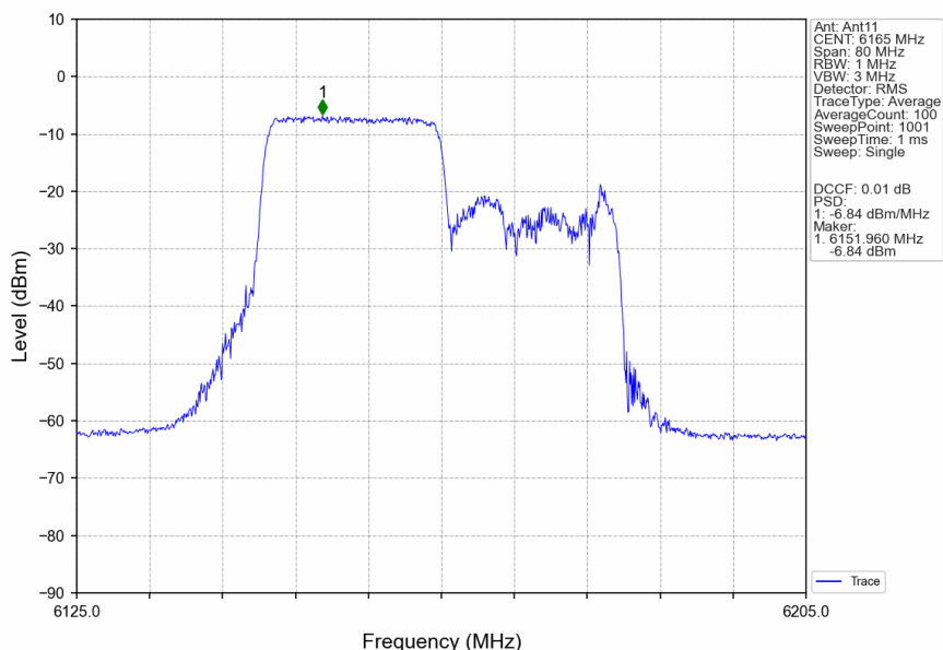
802.11ax(HEW40) MCH_6165MHz RU242 Left Ant11 NTN
