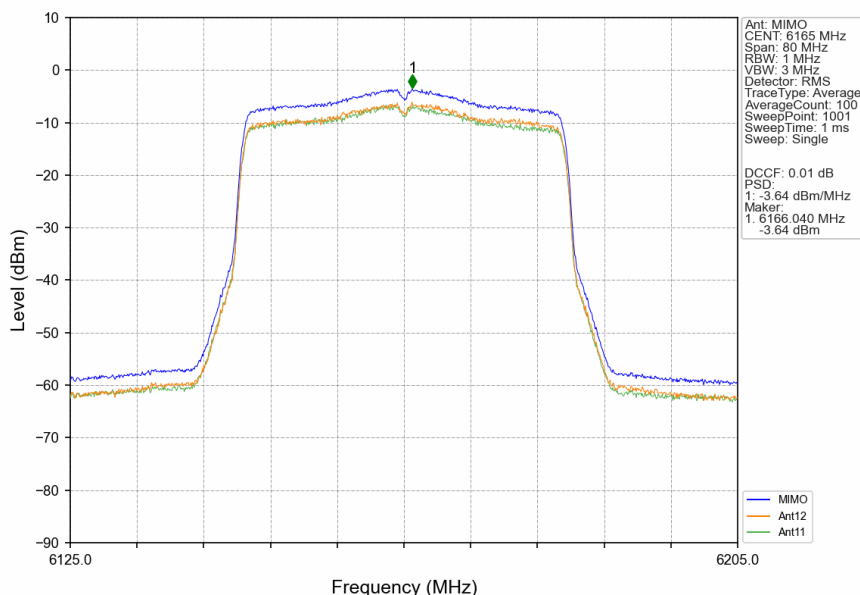
802.11ax(HEW40) MCH 6165MHz RU484 Left MIMO NTN
