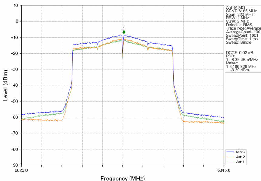
802.11ax(HEW160) MCH 6185MHz 2xRU996 Left MIMO NTNV
