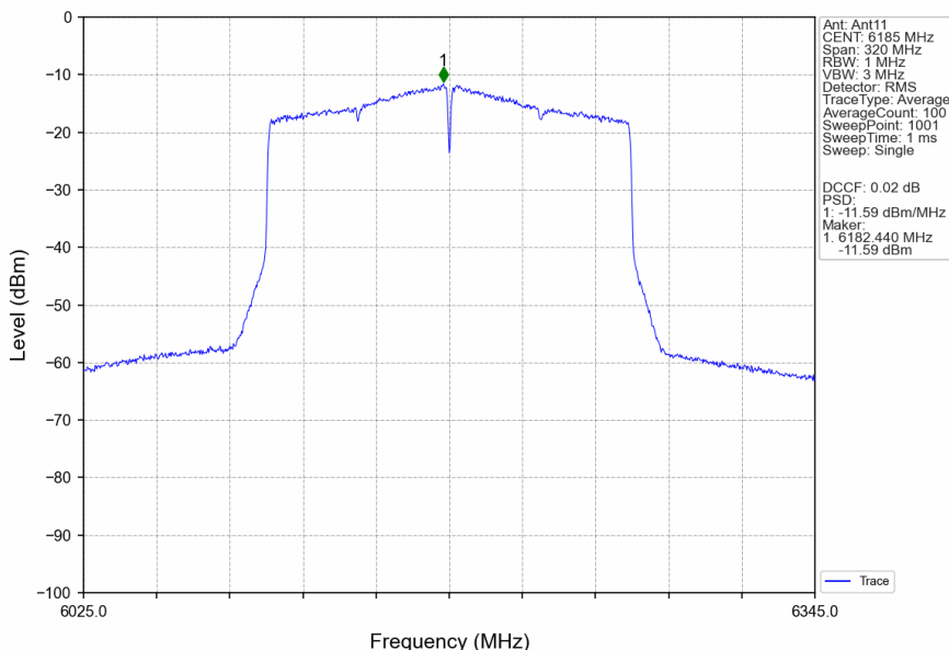
802.11ax(HEW160) MCH 6185MHz 2xRU996 Left MIMO NTNV
