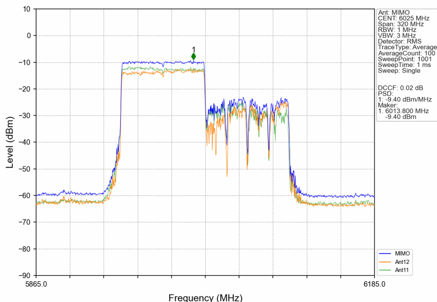
802.11ax(HEW160) LCH 6025MHz 2xRU996 Left Ant12 NTN
