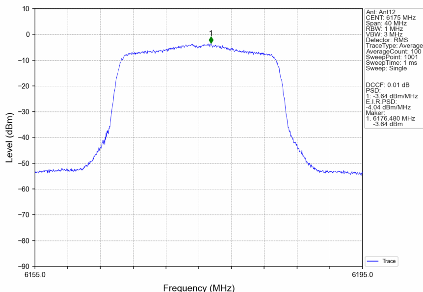
802.11ax(HEW20) MCH_6175MHz RU242 Left Ant12 NTN
