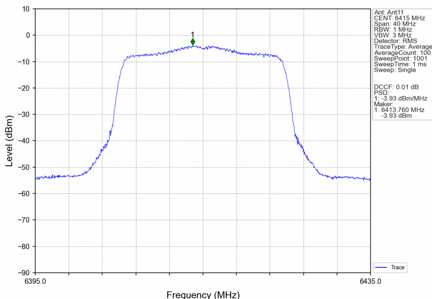
802.11ax(HEW20) HCH 6415MHz RU242 Left MIMO NTN
