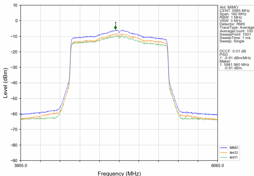
802.11ax(HEW80) LCH 5985MHz RU996 Left MIMO NTN
