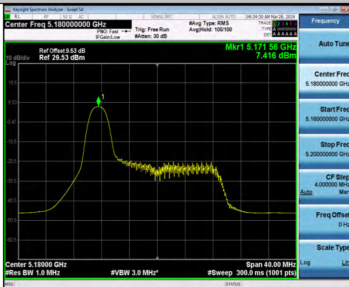
11AX20MIMO_Ant1_5180_52Tone_RU37
