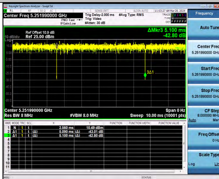
11AX20MIMO_Ant2_5260_52Tone_RU37
