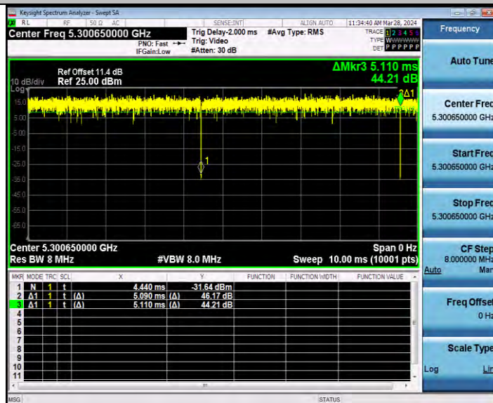
11AX20MIMO_Ant2_5300_52Tone_RU38
