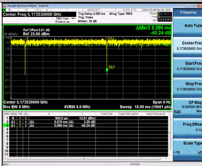
11AX20MIMO_Ant1_5180_106Tone_RU53
