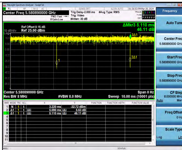
11AX20MIMO_Ant1_5580_52Tone_RU38
