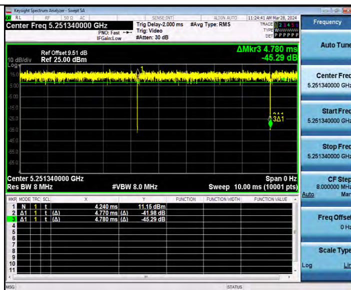
11AX20MIMO_Ant2_5260_26Tone_RU0
