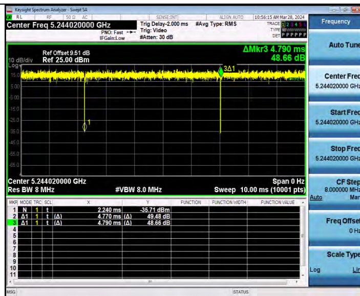
11AX20MIMO_Ant2_5240_26Tone_RU8
