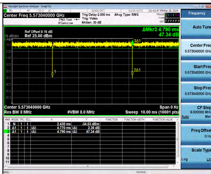
11AX20MIMO_Ant2_5580_26Tone_RU4
