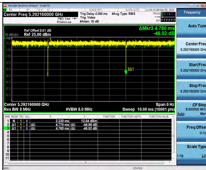
11AX20MIMO_Ant2_5300_26Tone_RU4
