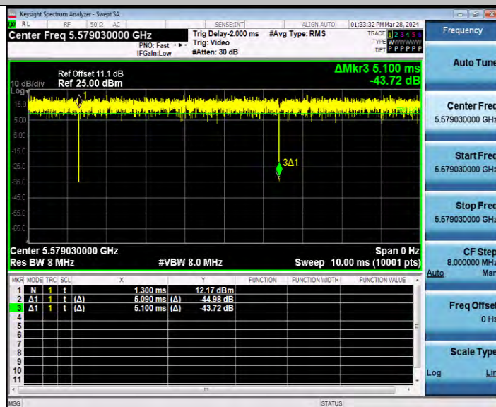
11AX20MIMO_Ant2_5580_52Tone_RU38
