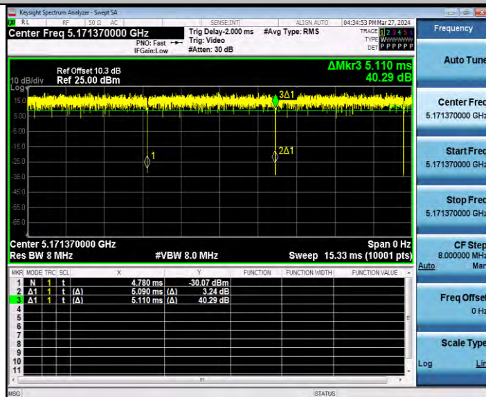
11AX20MIMO_Ant2_5180_52Tone_RU37
