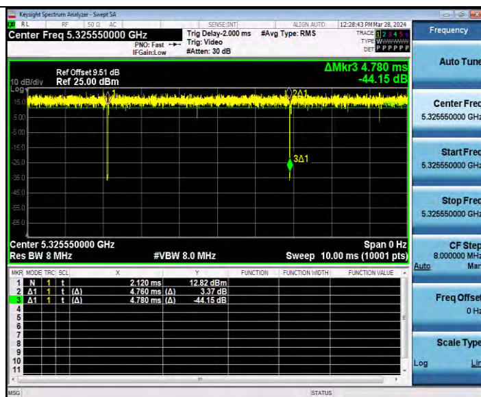
11AX20MIMO_Ant2_5320_26Tone_RU8
