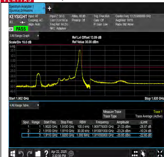
Band2-5MHz-QPSK-18625-1RB#0-PASS
