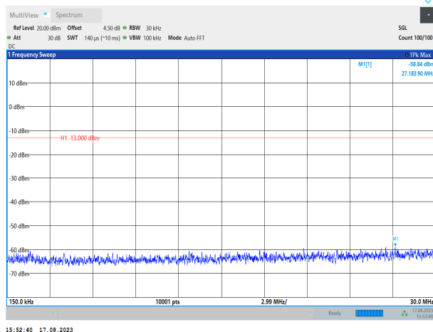
GSM850-128-0.15~30MHz
