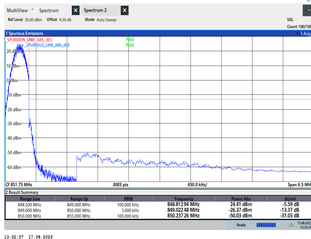
GSM850-251
