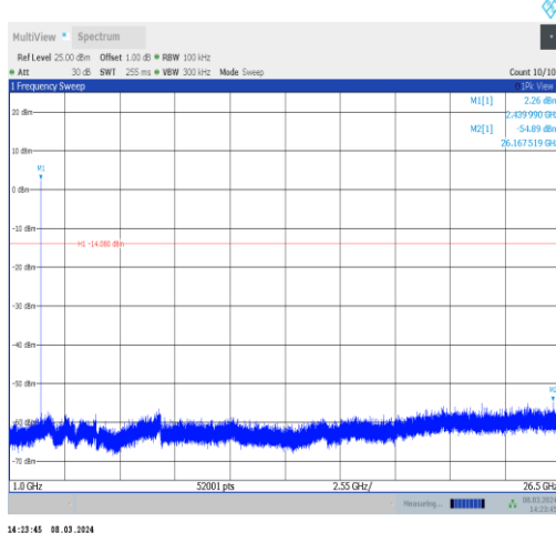
BLE_2M-Ant10-2440-1000~26500-PASS
