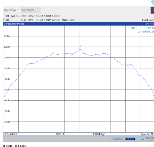
BLE_2M-Ant10-2478-0~Reference-PASS
