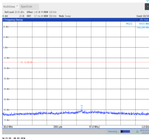
BLE_2M-Ant10-2404-30~1000-PASS
