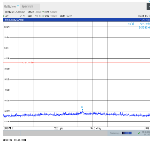
BLE_2M-Ant10-2440-30~1000-PASS
