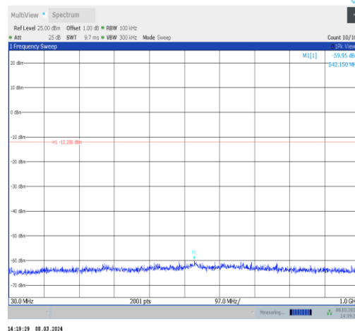
BLE_1M-Ant10-2480-30~1000-PASS
