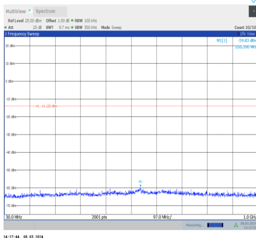
BLE_1M-Ant10-2440-30~1000-PASS
